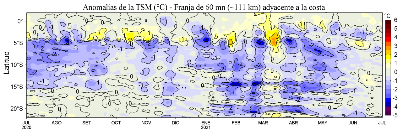
Figura 4. Variación promedio de las anomalías de la temperatura superficial del mar (TSM, °C) para una franja de 60 m.n. (~111 km) adyacente al litoral peruano para los últimos doce meses al 01 de julio de 2021. Datos: OSTIA-UKMO-L4-GLOB-v2.0 (UK Met. Office, 2012; Donlon et al, 2012) disponible en https://podaac.jpl.nasa.gov/dataset/OSTIA-UKMO-L4-GLOB-v2.0 . Las anomalías se calcularon con respecto al periodo 2007-2016.
