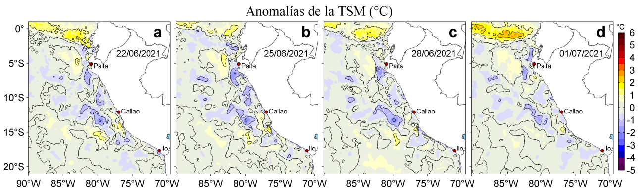
Figura 3. Anomalías de la temperatura superficial del mar (TSM, °C) para los días: a) 22, b) 25 y c) 28 de junio y d) 01 de julio de 2021. Las anomalías se calcularon respecto de la climatología para el periodo 2007-2016. Datos: OSTIA-UKMO-L4-GLOB-v2.0 (UK Met Office, 2012; Donlon et al, 2012).
