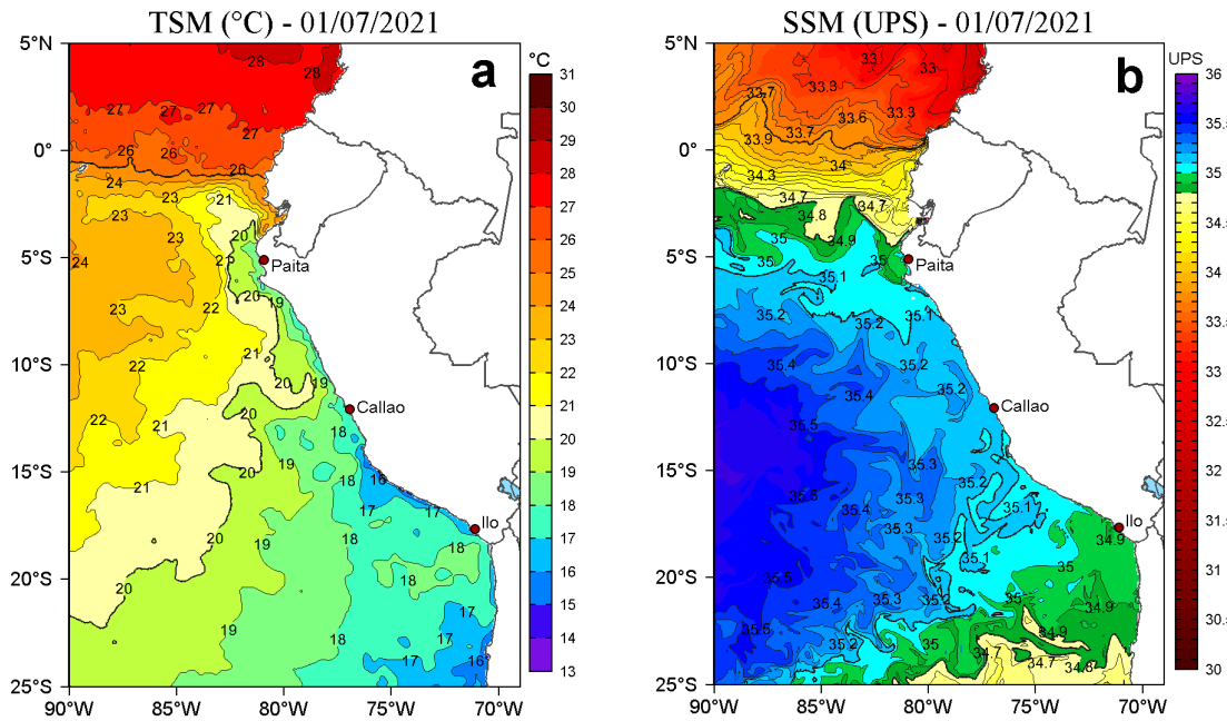
Figura 2. a) Temperatura superficial del mar (TSM, °C) y b) Salinidad superficial del mar (SSM) para el 01 de julio de 2021. Datos: OSTIA-UKMO-L4-GLOB-v2.0 (UK Met Office, 2012; Donlon et al, 2012) disponible en https://podaac.jpl.nasa.gov/dataset/OSTIA-UKMO-L4-GLOB-v2.0 para (a) y Hybrid Coordinate Ocean Model v. GOF5 3.1 (HYCOM; Halliwell et al., 1998; 2000; Bleck, 2001) para (b).
