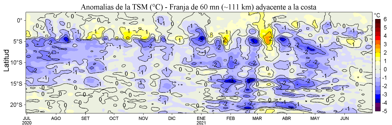
Figura 4. Variación promedio de las anomalías de la temperatura superficial del mar (TSM, °C) para una franja de 60 m.n. (~111 km) adyacente al litoral peruano para los últimos doce meses al 30 de junio de 2021. Datos: OSTIA-UKMO-L4-GLOB-v2.0 (UK Met. Office, 2012; Donlon et al, 2012) disponible en https://podaac.jpl.nasa.gov/dataset/OSTIA-UKMO-L4-GLOB-v2.0 . Las anomalías se calcularon con respecto al periodo 2007-2016.
