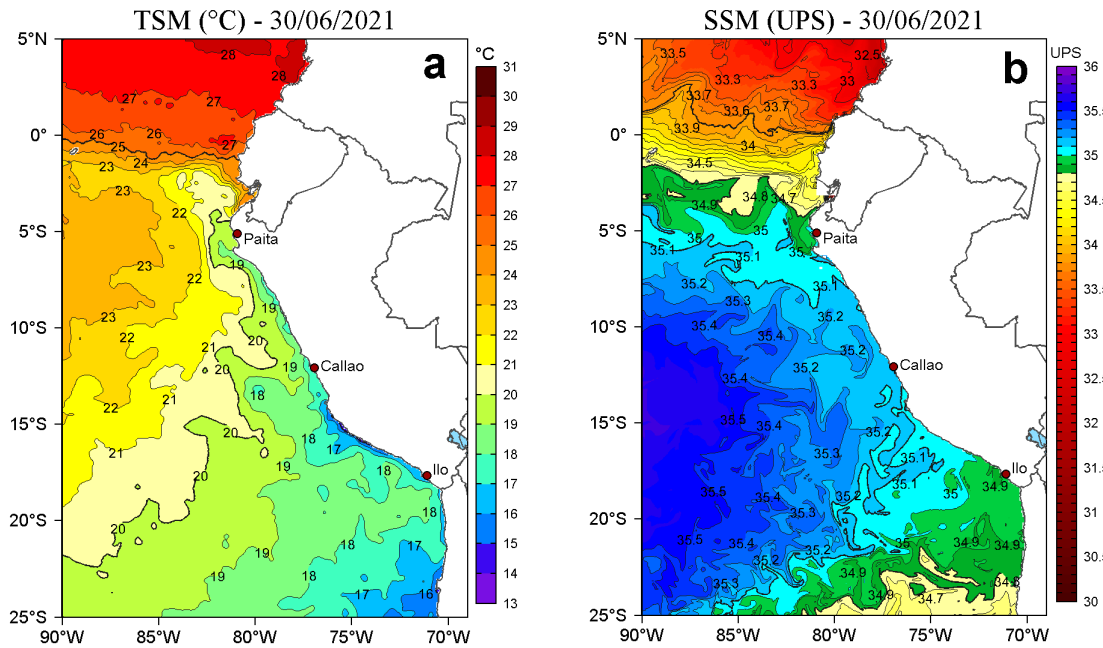
Figura 2. a) Temperatura superficial del mar (TSM, °C) y b) Salinidad superficial del mar (SSM) para el 30 de junio de 2021. Datos: OSTIA-UKMO-L4-GLOB-v2.0 (UK Met Office, 2012; Donlon et al, 2012) disponible en https://podaac.jpl.nasa.gov/dataset/OSTIA-UKMO-L4-GLOB-v2.0 para (a) y Hybrid Coordinate Ocean Model v. GOFS 3.1 (HYCOM; Halliwell et al., 1998; 2000; Bleck, 2001) para (b).
