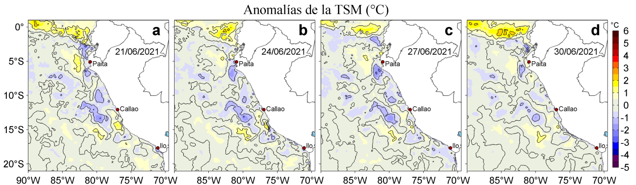
Figura 3. Anomalías de la temperatura superficial del mar (TSM, °C) para los días: a) 21, b) 24, c) 27 y d) 30 de junio de 2021. Las anomalías se calcularon respecto de la climatología para el periodo 2007-2016. Datos: OSTIA-UKMO-L4-GLOB-v2.0 (UK Met Office, 2012; Donlon et al, 2012).
