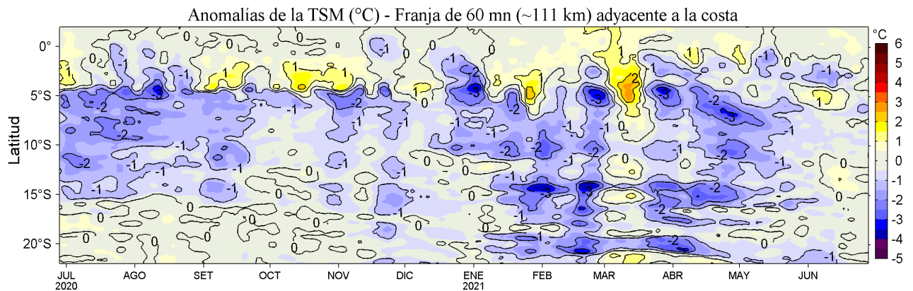
Figura 4. Variación promedio de las anomalías de la temperatura superficial del mar (TSM, °C) para una franja de 60 m.n. (~111 km) adyacente al litoral peruano para los últimos doce meses al 28 de junio de 2021. Datos: OSTIA-UKMO-L4-GLOB-v2.0 (UK Met. Office, 2012; Donlon et al, 2012) disponible en https://podaac.jpl.nasa.gov/dataset/OSTIA-UKMO-L4-GLOB-v2.0 . Las anomalías se calcularon con respecto al periodo 2007-2016.
