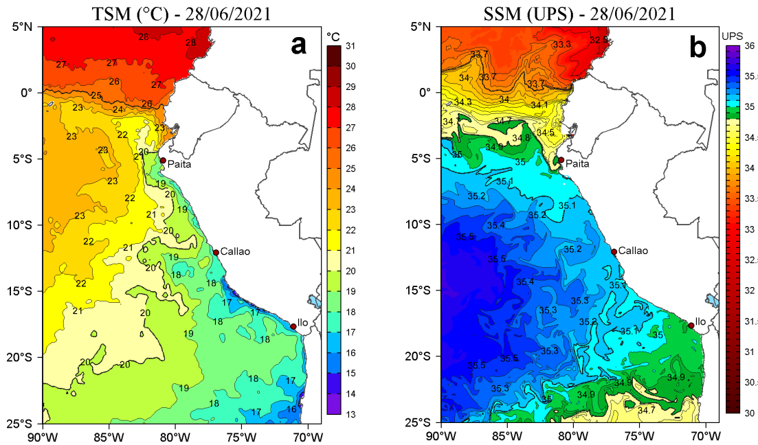
Figura 2. a) Temperatura superficial del mar (TSM, °C) y b) Salinidad superficial del mar (SSM) para el 28 de junio de 2021. Datos: OSTIA-UKMO-L4-GLOB-v2.0 (UK Met Office, 2012; Donlon et al, 2012) disponible en https://podaac.jpl.nasa.gov/dataset/OSTIA-UKMO-L4-GLOB-v2.0 para (a) y Hybrid Coordinate Ocean Model v. GOFS 3.1 (HYCOM; Halliwell et al., 1998; 2000; Bleck, 2001) para (b).
