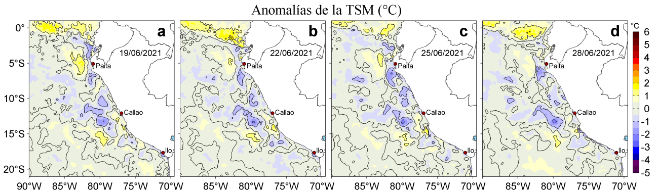
Figura 3. Anomalías de la temperatura superficial del mar (TSM, °C) para los días: a) 19, b) 22, c) 25 y d) 28 de junio de 2021. Las anomalías se calcularon respecto de la climatología para el periodo 2007-2016. Datos: OSTIA-UKMO-L4-GLOB-v2.0 (UK Met Office, 2012; Donlon et al, 2012).
