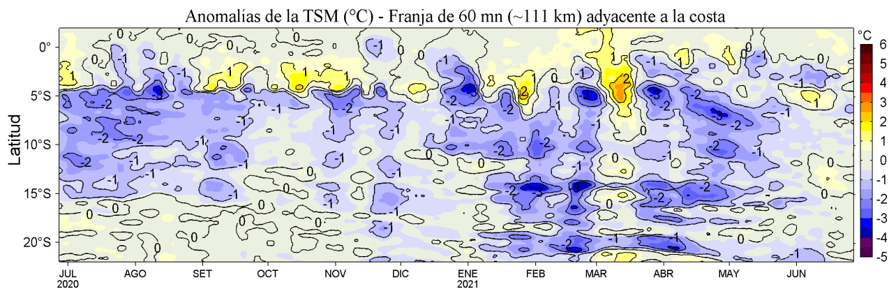
Figura 4. Variación promedio de las anomalías de la temperatura superficial del mar (TSM, °C) para una franja de 60 m.n. (~111 km) adyacente al litoral peruano para los últimos doce meses al 27 de junio de 2021. Datos: OSTIA-UKMO-L4-GLOB-v2.0 (UK Met. Office, 2012; Donlon et al, 2012) disponible en https://podaac.jpl.nasa.gov/dataset/OSTIA-UKMO-L4-GLOB-v2.0 . Las anomalías se calcularon con respecto al periodo 2007-2016.
