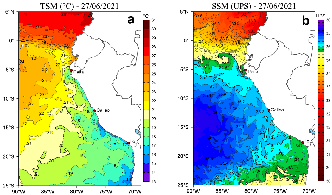
Figura 2. a) Temperatura superficial del mar (TSM, °C) y b) Salinidad superficial del mar (SSM) para el 27 de junio de 2021. Datos: OSTIA-UKMO-L4-GLOB-v2.0 (UK Met Office, 2012; Donlon et al, 2012) disponible en https://podaac.jpl.nasa.gov/dataset/OSTIA-UKMO-L4-GLOB-v2.0 para (a) y Hybrid Coordinate Ocean Model v. GOFS 3.1 (HYCOM; Halliwell et al., 1998; 2000; Bleck, 2001) para (b).
