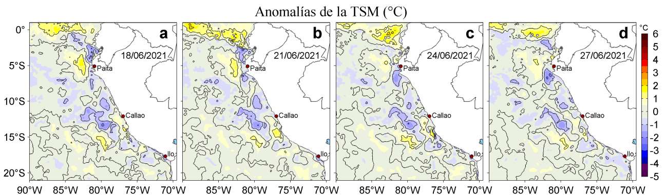
Figura 3. Anomalías de la temperatura superficial del mar (TSM, °C) para los días: a) 18, b) 21, c) 24 y d) 27 de junio de 2021. Las anomalías se calcularon respecto de la climatología para el periodo 2007-2016. Datos: OSTIA-UKMO-L4-GLOB-v2.0 (UK Met Office, 2012; Donlon et al, 2012).
