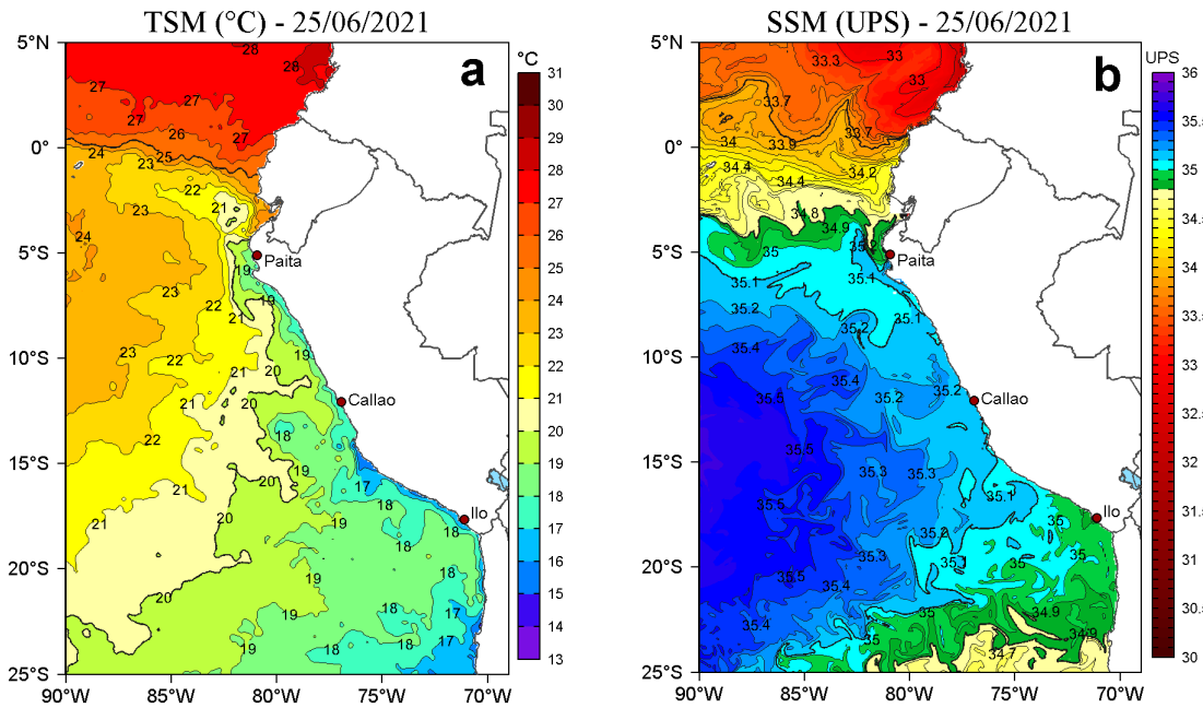
Figura 2. a) Temperatura superficial del mar (TSM, °C) y b) Salinidad superficial del mar (SSM) para el 25 de junio de 2021. Datos: OSTIA-UKMO-L4-GLOB-v2.0 (UK Met Office, 2012; Donlon et al, 2012) disponible en https://podaac.jpl.nasa.gov/dataset/OSTIA-UKMO-L4-GLOB-v2.0 para (a) y Hybrid Coordinate Ocean Model v. GOFS 3.1 (HYCOM; Halliwell et al., 1998; 2000; Bleck, 2001) para (b).
