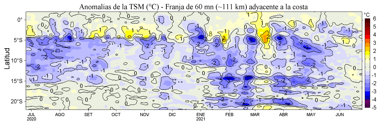
Figura 4. Variación promedio de las anomalías de la temperatura superficial del mar (TSM, °C) para una franja de 60 m.n. (~111 km) adyacente al litoral peruano para los últimos doce meses al 25 de junio de 2021. Datos: OSTIA-UKMO-L4-GLOB-v2.0 (UK Met. Office, 2012; Donlon et al, 2012) disponible en https://podaac.jpl.nasa.gov/dataset/OSTIA-UKMO-L4-GLOB-v2.0 . Las anomalías se calcularon con respecto al periodo 2007-2016.
