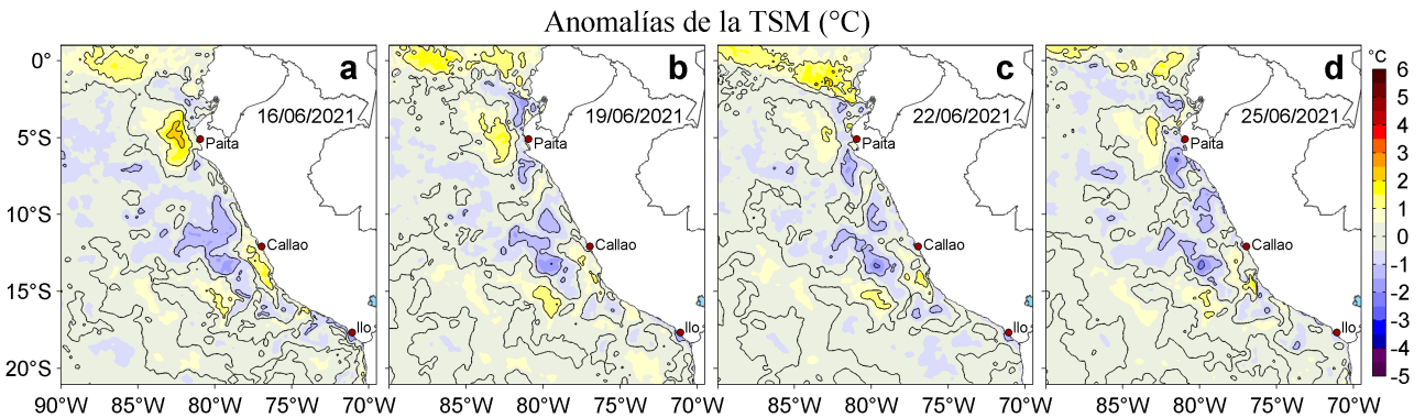
Figura 3. Anomalías de la temperatura superficial del mar (TSM, °C) para los días: a) 16, b) 19, c) 22 y d) 25 de junio de 2021. Las anomalías se calcularon respecto de la climatología para el periodo 2007-2016. Datos: OSTIA-UKMO-L4-GLOB-v2.0 (UK Met Office, 2012; Donlon et al, 2012).
