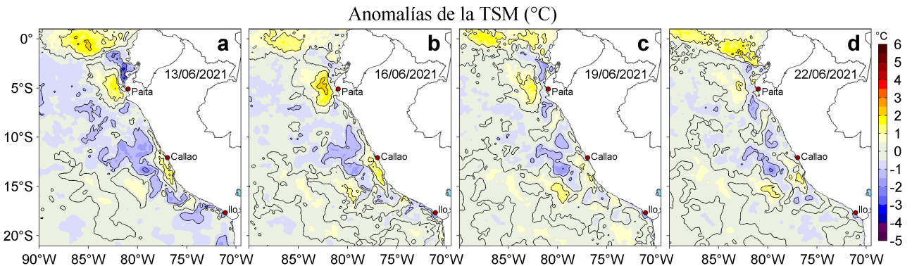
Figura 3. Anomalías de la temperatura superficial del mar (TSM, °C) para los días: a) 13, b) 16, c) 19 y d) 22 de junio de 2021. Las anomalías se calcularon respecto de la climatología para el periodo 2007-2016. Datos: OSTIA-UKMO-L4-GLOB-v2.0 (UK Met Office, 2012; Donlon et al, 2012).
