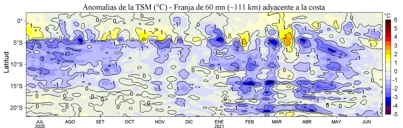
Figura 4. Variación promedio de las anomalías de la temperatura superficial del mar (TSM, °C) para una franja de 60 mn (~111 km) adyacente al litoral peruano para los últimos doce meses al 17 de junio de 2021. Datos: OSTIA-UKMO-L4-GLOB-v2.0 (UK Met. Office, 2012; Donlon et al, 2012) disponible en https://podaac.jpl.nasa.gov/dataset/OSTIA-UKMO-L4-GLOB-v2.0 . Las anomalías se calcularon con respecto al periodo 2007-2016.
