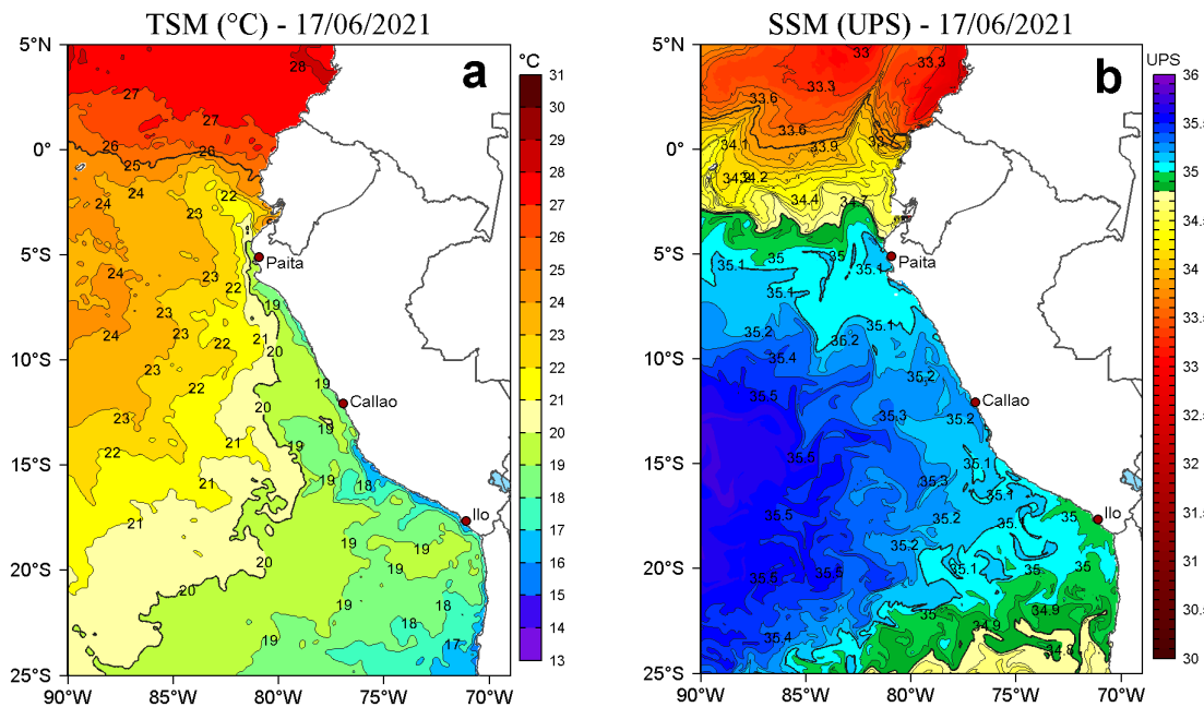
Figura 2. a) Temperatura superficial del mar (TSM, °C) y b) Salinidad superficial del mar (SSM) para el 17 de junio de 2021. Datos: OSTIA-UKMO-L4-GLOB-v2.0 (UK Met Office, 2012; Donlon et al, 2012) disponible en https://podaac.jpl.nasa.gov/dataset/OSTIA-UKMO-L4-GLOB-v2.0 para (a) y Hybrid Coordinate Ocean Model v. GOFS 3.1 (HYCOM; Halliwell et al., 1998; 2000; Bleck, 2001) para (b).
