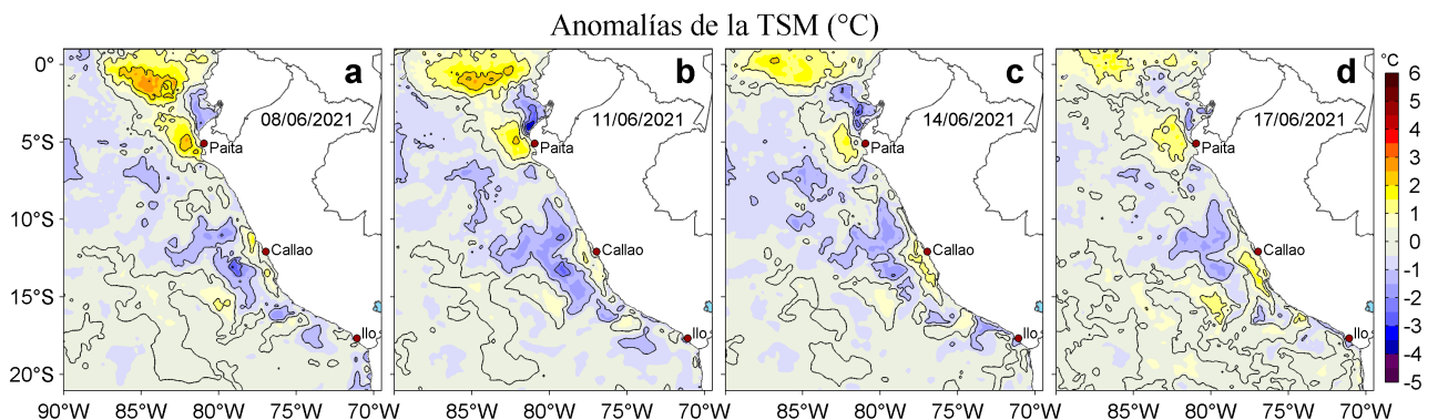
Figura 3. Anomalías de la temperatura superficial del mar (TSM, °C) para los días: a) 08, b) 11, c) 14 y d) 17 de junio de 2021. Las anomalías se calcularon respecto de la climatología para el periodo 2007-2016. Datos: OSTIA-UKMO-L4-GLOB-v2.0 (UK Met Office, 2012; Donlon et al, 2012).
