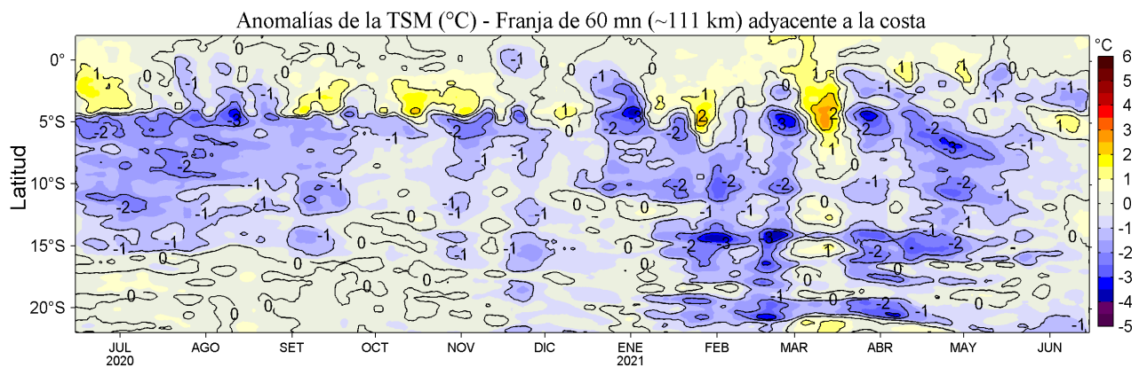
Figura 4. Variación promedio de las anomalías de la temperatura superficial del mar (TSM, °C) para una franja de 60 mn (~111 km) adyacente al litoral peruano para los últimos doce meses al 15 de junio de 2021. Datos: OSTIA-UKMO-L4-GLOB-v2.0 (UK Met. Office, 2012; Donlon et al, 2012) disponible en https://podaac.jpl.nasa.gov/dataset/OSTIA-UKMO-L4-GLOB-v2.0 . Las anomalías se calcularon con respecto al periodo 2007-2016.
