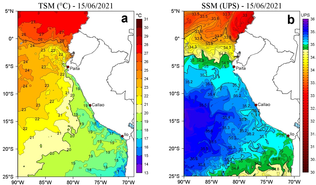
Figura 2. a) Temperatura superficial del mar (TSM, °C) y b) Salinidad superficial del mar (SSM) para el 15 de junio de 2021. Datos: OSTIA-UKMO-L4-GLOB-v2.0 (UK Met Office, 2012; Donlon et al, 2012) disponible en https://podaac.jpl.nasa.gov/dataset/OSTIA-UKMO-L4-GLOB-v2.0 para (a) y Hybrid Coordinate Ocean Model v. GOFS 3.1 (HYCOM; Halliwell et al., 1998; 2000; Bleck, 2001) para (b).
