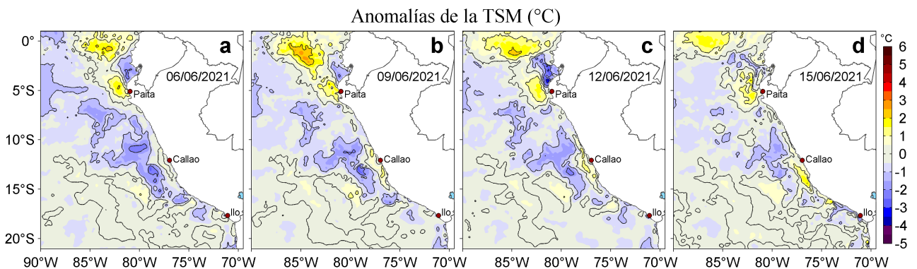
Figura 3. Anomalías de la temperatura superficial del mar (TSM, °C) para los días: a) 06, b) 09, c) 12 y d) 15 de junio de 2021. Las anomalías se calcularon respecto de la climatología para el periodo 2007-2016. Datos: OSTIA-UKMO-L4-GLOB-v2.0 (UK Met Office, 2012; Donlon et al, 2012).
