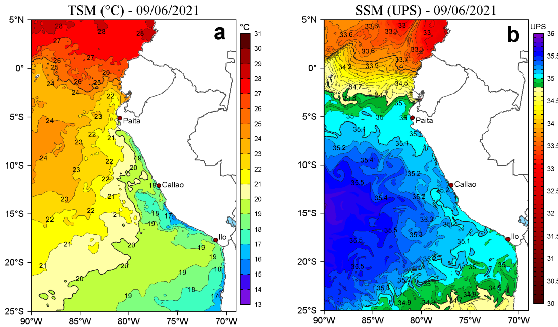
Figura 2. a) Temperatura superficial del mar (TSM, °C) y b) Salinidad superficial del mar (SSM) para el 09 de junio de 2021. Datos: OSTIA-UKMO-L4-GLOB-v2.0 (UK Met Office, 2012; Donlon et al, 2012) disponible en https://podaac.jpl.nasa.gov/dataset/OSTIA-UKMO-L4-GLOB-v2.0 para (a) y Hybrid Coordinate Ocean Model v. GOFS 3.1 (HYCOM; Halliwell et al., 1998; 2000; Bleck, 2001) para (b).
