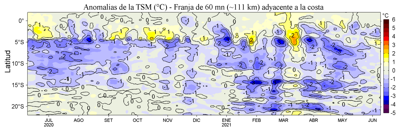
Figura 4. Variación promedio de las anomalías de la temperatura superficial del mar (TSM, °C) para una franja de 60 mn (~111 km) adyacente al litoral peruano para los últimos doce meses al 09 de junio de 2021. Datos: OSTIA-UKMO-L4-GLOB-v2.0 (UK Met. Office, 2012; Donlon et al, 2012) disponible en https://podaac.jpl.nasa.gov/dataset/OSTIA-UKMO-L4-GLOB-v2.0 . Las anomalías se calcularon con respecto al periodo 2007-2016.
