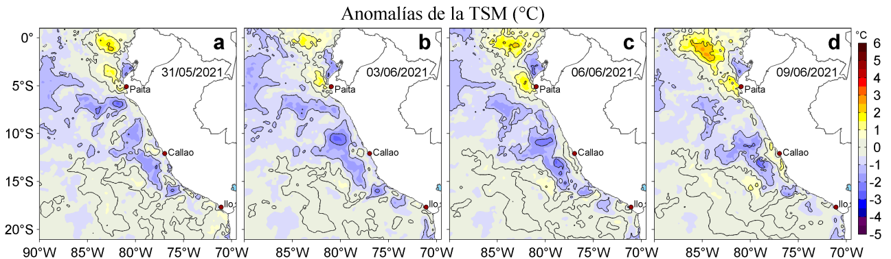
Figura 3. Anomalías de la temperatura superficial del mar (TSM, °C) para los días: a) 31 de mayo, b) 03, c) 06 y d) 09 de junio de 2021. Las anomalías se calcularon respecto de la climatología para el periodo 2007-2016. Datos: OSTIA-UKMO-L4-GLOB-v2.0 (UK Met Office, 2012; Donlon et al, 2012).
