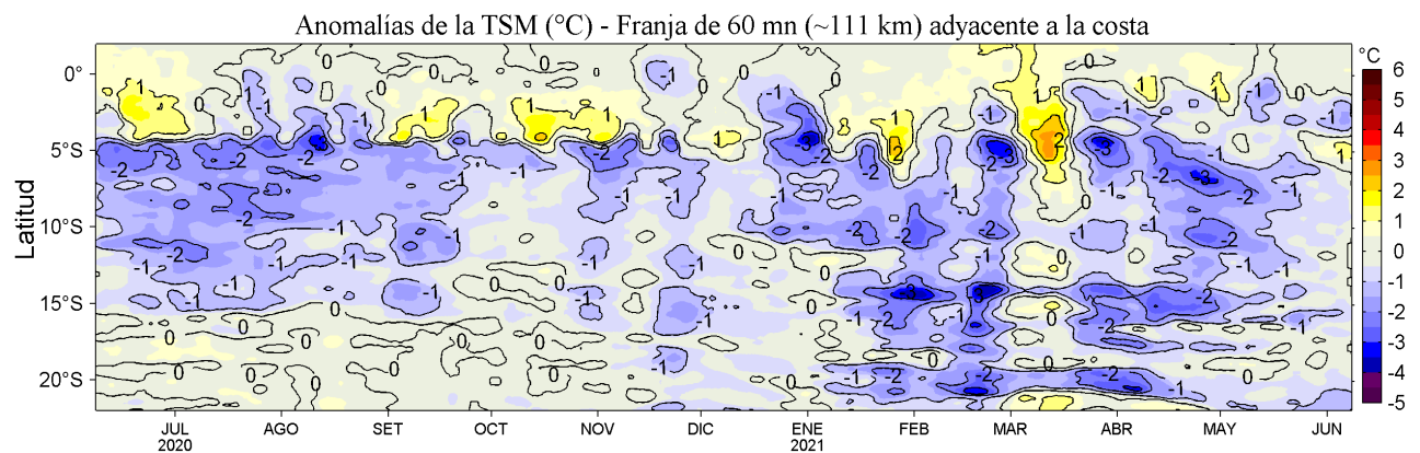
Figura 4. Variación promedio de las anomalías de la temperatura superficial del mar (TSM, °C) para una franja de 60 mn (~111 km) adyacente al litoral peruano para los últimos doce meses al 08 de junio de 2021. Datos: OSTIA-UKMO-L4-GLOB-v2.0 (UK Met. Office, 2012; Donlon et al, 2012) disponible en https://podaac.jpl.nasa.gov/dataset/OSTIA-UKMO-L4-GLOB-v2.0 . Las anomalías se calcularon con respecto al periodo 2007-2016.
