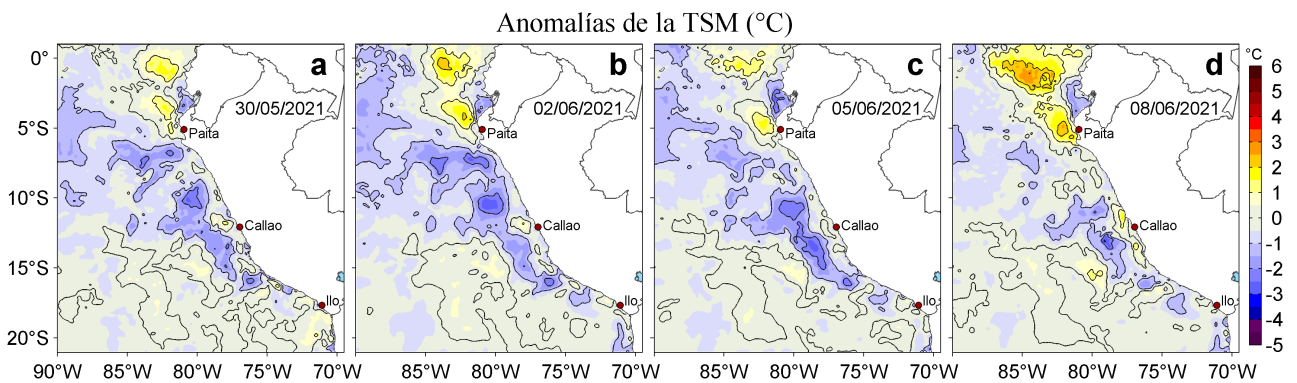
Figura 3. Anomalías de la temperatura superficial del mar (TSM, °C) para los días: a) 30 de mayo, b) 02, c) 05 y d) 08 de junio de 2021. Las anomalías se calcularon respecto de la climatología para el periodo 2007-2016. Datos: OSTIA-UKMO-L4-GLOB-v2.0 (UK Met Office, 2012; Donlon et al, 2012).
