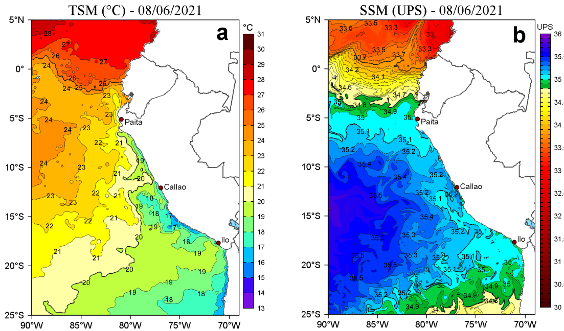
Figura 2. a) Temperatura superficial del mar (TSM, °C) y b) Salinidad superficial del mar (SSM) para el 08 de junio de 2021. Datos: OSTIA-UKMO-L4-GLOB-v2.0 (UK Met Office, 2012; Donlon et al, 2012) disponible en https://podaac.jpl.nasa.gov/dataset/OSTIA-UKMO-L4-GLOB-v2.0 para (a) y Hybrid Coordinate Ocean Model v. GOFS 3.1 (HYCOM; Halliwell et al., 1998; 2000; Bleck, 2001) para (b).
