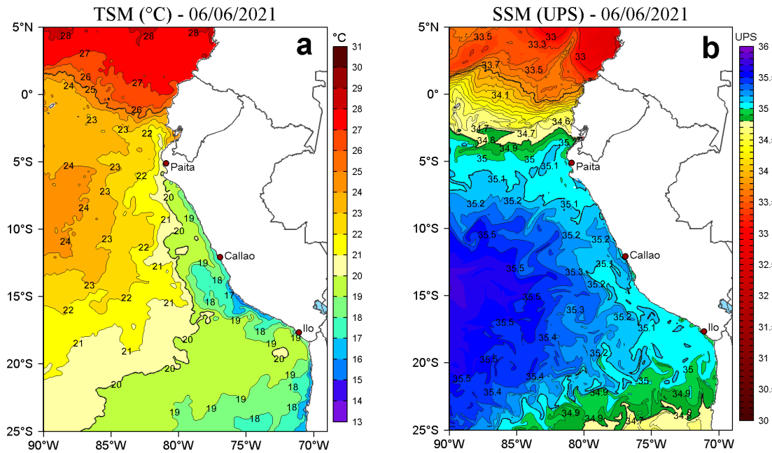
Figura 2. a) Temperatura superficial del mar (TSM, °C) y b) Salinidad superficial del mar (SSM) para el 06 de junio de 2021. Datos: OSTIA-UKMO-L4-GLOB-v2.0 (UK Met Office, 2012; Donlon et al, 2012) disponible en https://podaac.jpl.nasa.gov/dataset/OSTIA-UKMO-L4-GLOB-v2.0 para (a) y Hybrid Coordinate Ocean Model v. GOFS 3.1 (HYCOM; Halliwell et al., 1998; 2000; Bleck, 2001) para (b).
