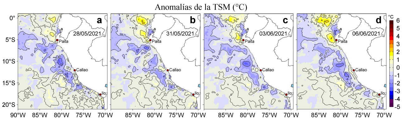
Figura 3. Anomalías de la temperatura superficial del mar (TSM, °C) para los días: a) 28 y b) 31 de mayo, c) 03 y d) 06 de junio de 2021. Las anomalías se calcularon respecto de la climatología para el periodo 2007-2016. Datos: OSTIA-UKMO-L4-GLOB-v2.0 (UK Met Office, 2012; Donlon et al, 2012).
