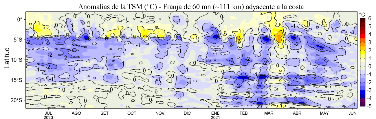
Figura 4. Variación promedio de las anomalías de la temperatura superficial del mar (TSM, °C) para una franja de 60 mn (~111 km) adyacente al litoral peruano para los últimos doce meses al 06 de junio de 2021. Datos: OSTIA-UKMO-L4-GLOB-v2.0 (UK Met. Office, 2012; Donlon et al, 2012) disponible en https://podaac.jpl.nasa.gov/dataset/OSTIA-UKMO-L4-GLOB-v2.0 . Las anomalías se calcularon con respecto al periodo 2007-2016.
