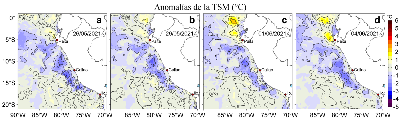
Figura 3. Anomalías de la temperatura superficial del mar (TSM, °C) para los días: a) 26 y b) 29 de mayo, c) 01 y d) 04 de junio de 2021. Las anomalías se calcularon respecto de la climatología para el periodo 2007-2016. Datos: OSTIA-UKMO-L4-GLOB-v2.0 (UK Met Office, 2012; Donlon et al, 2012).
