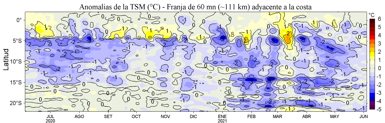
Figura 4. Variación promedio de las anomalías de la temperatura superficial del mar (TSM, °C) para una franja de 60 m.n. (~111 km) adyacente al litoral peruano para los últimos doce meses al 04 de junio de 2021. Datos: OSTIA-UKMO-L4-GLOB-v2.0 (UK Met. Office, 2012; Donlon et al, 2012) disponible en https://podaac.jpl.nasa.gov/dataset/OSTIA-UKMO-L4-GLOB-v2.0 . Las anomalías se calcularon con respecto al periodo 2007-2016.
