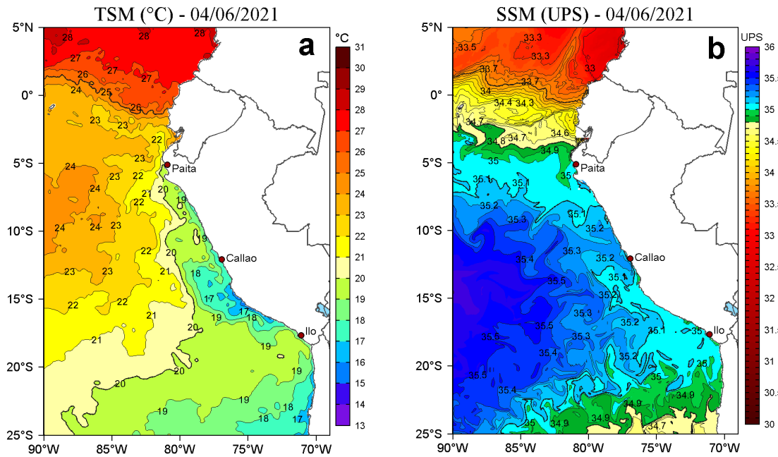
Figura 2. a) Temperatura superficial del mar (TSM, °C) y b) Salinidad superficial del mar (SSM) para el 04 de junio de 2021. Datos: OSTIA-UKMO-L4-GLOB-v2.0 (UK Met Office, 2012; Donlon et al, 2012) disponible en https://podaac.jpl.nasa.gov/dataset/OSTIA-UKMO-L4-GLOB-v2.0 para (a) y Hybrid Coordinate Ocean Model v. GOFS 3.1 (HYCOM; Halliwell et al., 1998; 2000; Bleck, 2001) para (b).
