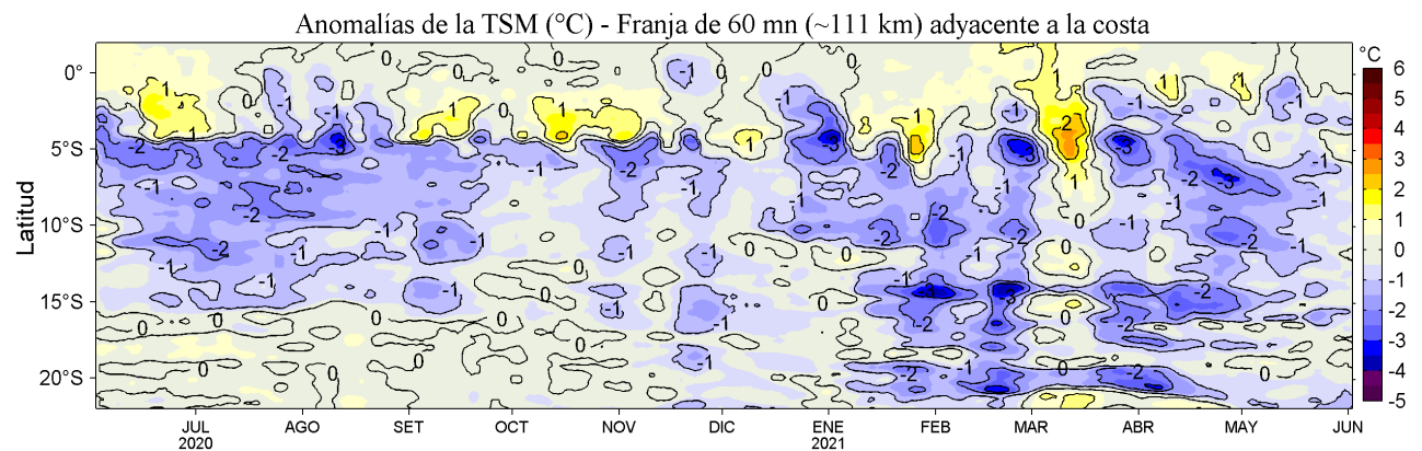
Figura 4. Variación promedio de las anomalías de la temperatura superficial del mar (TSM, °C) para una franja de 60 mn (~111 km) adyacente al litoral peruano para los últimos doce meses al 02 de junio de 2021. Datos: OSTIA-UKMO-L4-GLOB-v2.0 (UK Met. Office, 2012; Donlon et al, 2012) disponible en https://podaac.jpl.nasa.gov/dataset/OSTIA-UKMO-L4-GLOB-v2.0 . Las anomalías se calcularon con respecto al periodo 2007-2016.
