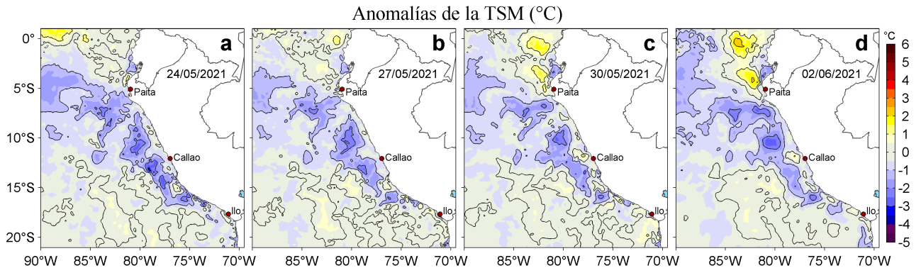
Figura 3. Anomalías de la temperatura superficial del mar (TSM, °C) para los días: a) 24, b) 27 y c) 30 de mayo y d) 02 de junio de 2021. Las anomalías se calcularon respecto de la climatología para el periodo 2007-2016. Datos: OSTIA-UKMO-L4-GLOB-v2.0 (UK Met Office, 2012; Donlon et al, 2012).
