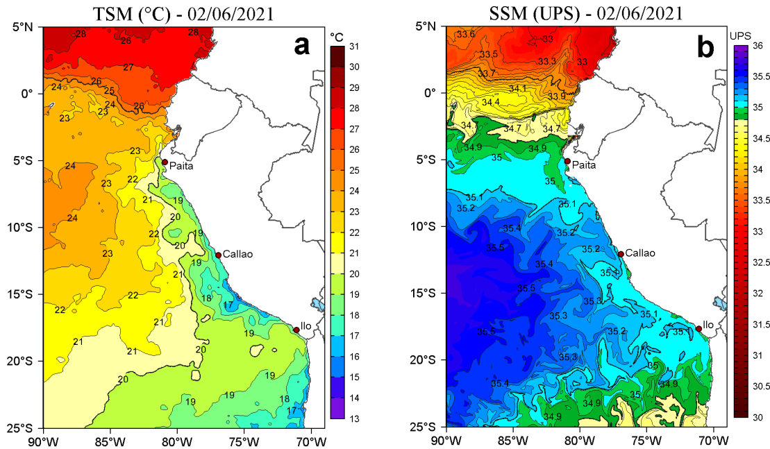
Figura 2. a) Temperatura superficial del mar (TSM, °C) y b) Salinidad superficial del mar (SSM) para el 02 de junio de 2021. Datos: OSTIA-UKMO-L4-GLOB-v2.0 (UK Met Office, 2012; Donlon et al, 2012) disponible en https://podaac.jpl.nasa.gov/dataset/OSTIA-UKMO-L4-GLOB-v2.0 para (a) y Hybrid Coordinate Ocean Model v. GOFS 3.1 (HYCOM; Halliwell et al., 1998; 2000; Bleck, 2001) para (b).
