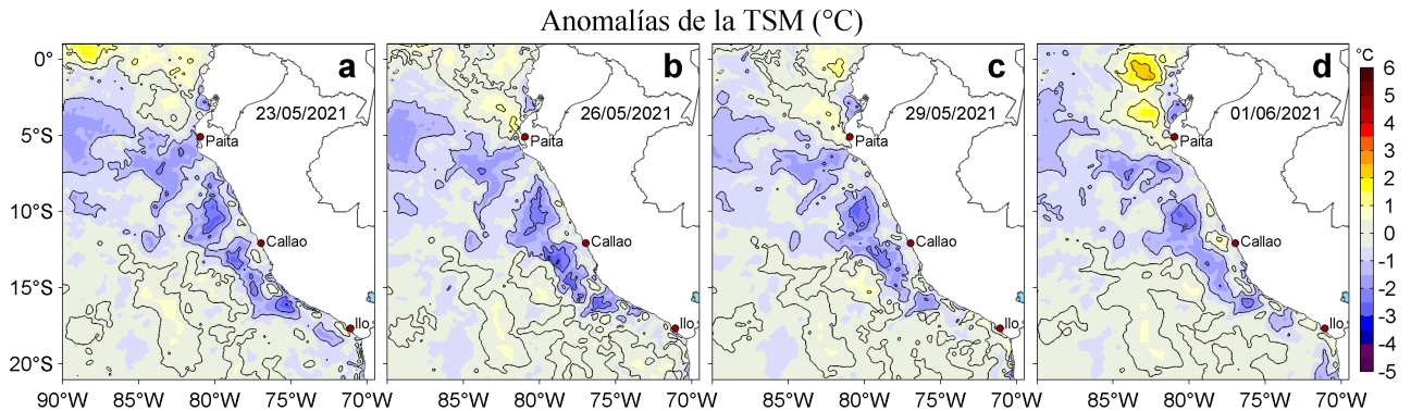
Figura 3. Anomalías de la temperatura superficial del mar (TSM, °C) para los días: a) 23, b) 26 y c) 29 de mayo y d) 01 de junio de 2021. Las anomalías se calcularon respecto de la climatología para el periodo 2007-2016. Datos: OSTIA-UKMO-L4-GLOB-v2.0 (UK Met Office, 2012; Donlon et al, 2012).
