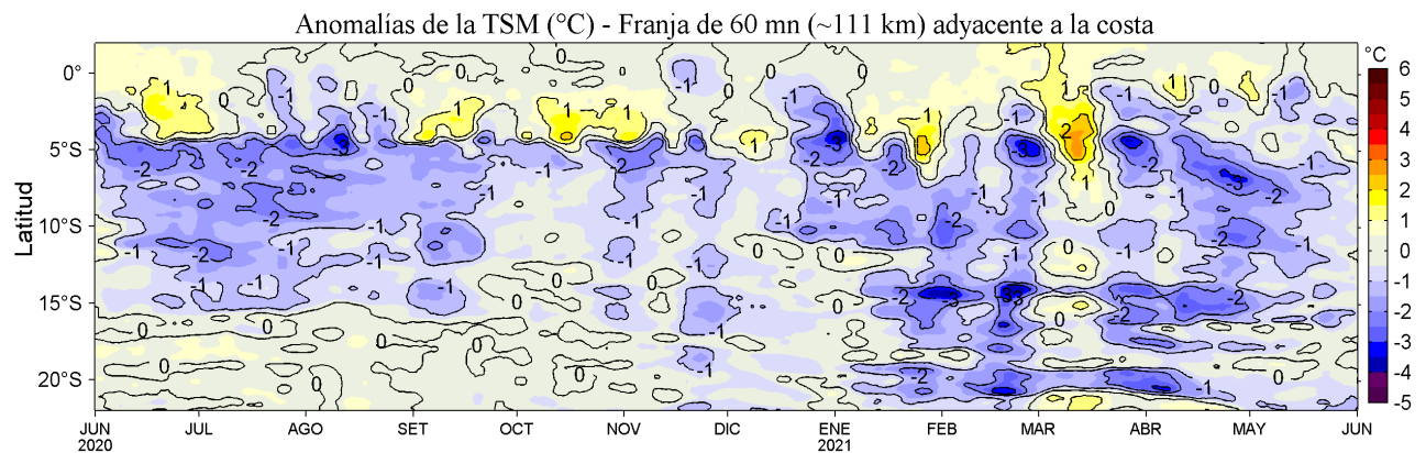
Figura 4. Variación promedio de las anomalías de la temperatura superficial del mar (TSM, °C) para una franja de 60 mn (~111 km) adyacente al litoral peruano para los últimos doce meses al 01 de junio de 2021. Datos: OSTIA-UKMO-L4-GLOB-v2.0 (UK Met. Office, 2012; Donlon et al, 2012) disponible en https://podaac.jpl.nasa.gov/dataset/OSTIA-UKMO-L4-GLOB-v2.0 . Las anomalías se calcularon con respecto al periodo 2007-2016.
