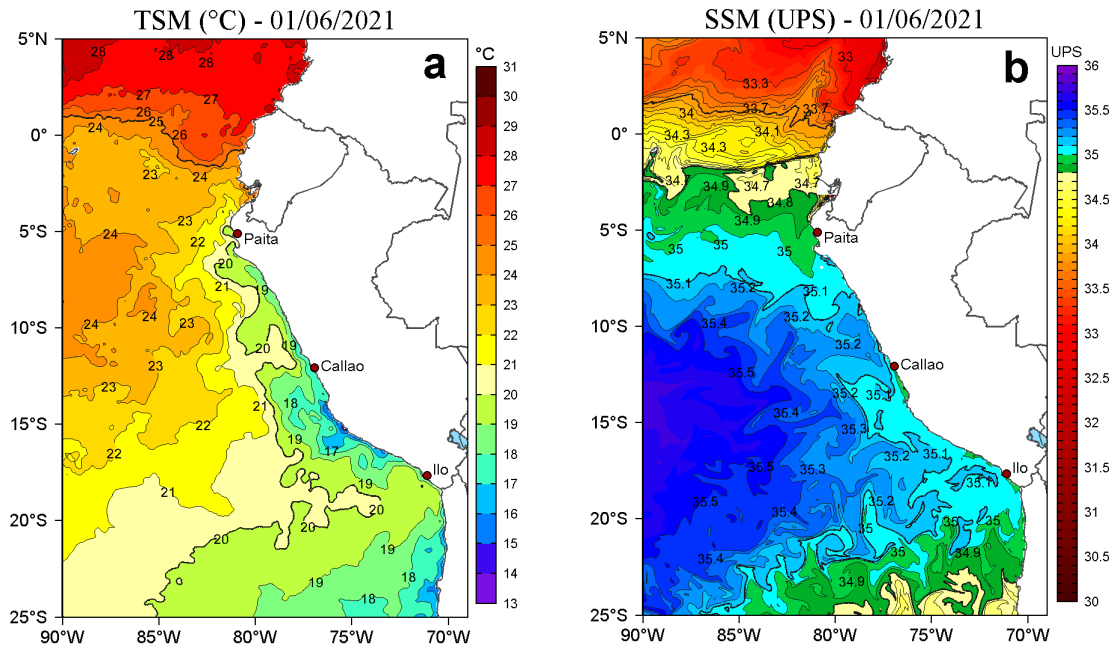
Figura 2. a) Temperatura superficial del mar (TSM, °C) y b) Salinidad superficial del mar (SSM) para el 01 de junio de 2021. Datos: OSTIA-UKMO-L4-GLOB-v2.0 (UK Met Office, 2012; Donlon et al, 2012) disponible en https://podaac.jpl.nasa.gov/dataset/OSTIA-UKMO-L4-GLOB-v2.0 para (a) y Hybrid Coordinate Ocean Model v. GOF5 3.1 (HYCOM; Halliwell et al., 1998; 2000; Bleck, 2001) para (b).
