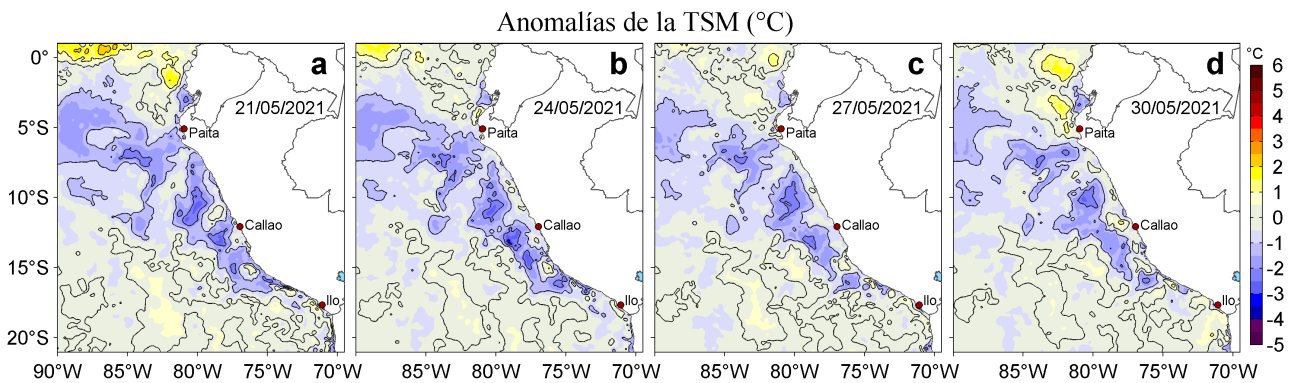
Figura 3. Anomalías de la temperatura superficial del mar (TSM, °C) para los días: a) 21, b) 24, c) 27 y d) 30 de mayo de 2021. Las anomalías se calcularon respecto de la climatología para el periodo 2007-2016. Datos: OSTIA-UKMO-L4-GLOB-v2.0 (UK Met Office, 2012; Donlon et al, 2012).
