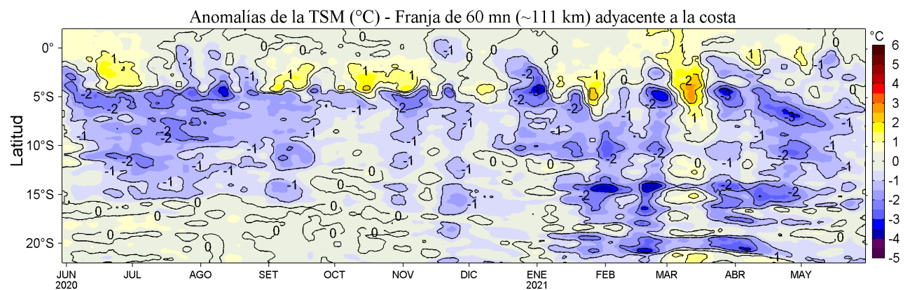
Figura 4. Variación promedio de las anomalías de la temperatura superficial del mar (TSM, °C) para una franja de 60 mn (~111 km) adyacente al litoral peruano para los últimos doce meses al 30 de mayo de 2021. Datos: OSTIA-UKMO-L4-GLOB-v2.0 (UK Met. Office, 2012; Donlon et al, 2012) disponible en https://podaac.jpl.nasa.gov/dataset/OSTIA-UKMO-L4-GLOB-v2.0 . Las anomalías se calcularon con respecto al periodo 2007-2016.
