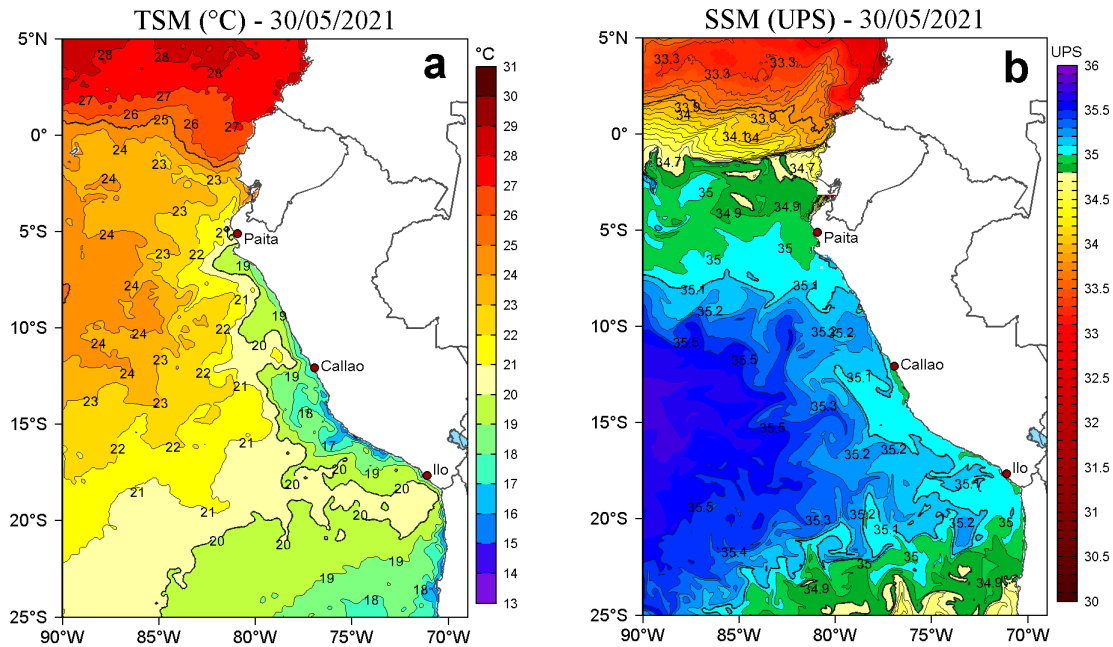
Figura 2. a) Temperatura superficial del mar (TSM, °C) y b) Salinidad superficial del mar (SSM) para el 30 de mayo de 2021. Datos: OSTIA-UKMO-L4-GLOB-v2.0 (UK Met Office, 2012; Donlon et al, 2012) disponible en https://podaac.jpl.nasa.gov/dataset/OSTIA-UKMO-L4-GLOB-v2.0 para (a) y Hybrid Coordinate Ocean Model v. GOFS 3.1 (HYCOM; Halliwell et al., 1998; 2000; Bleck, 2001) para (b).
