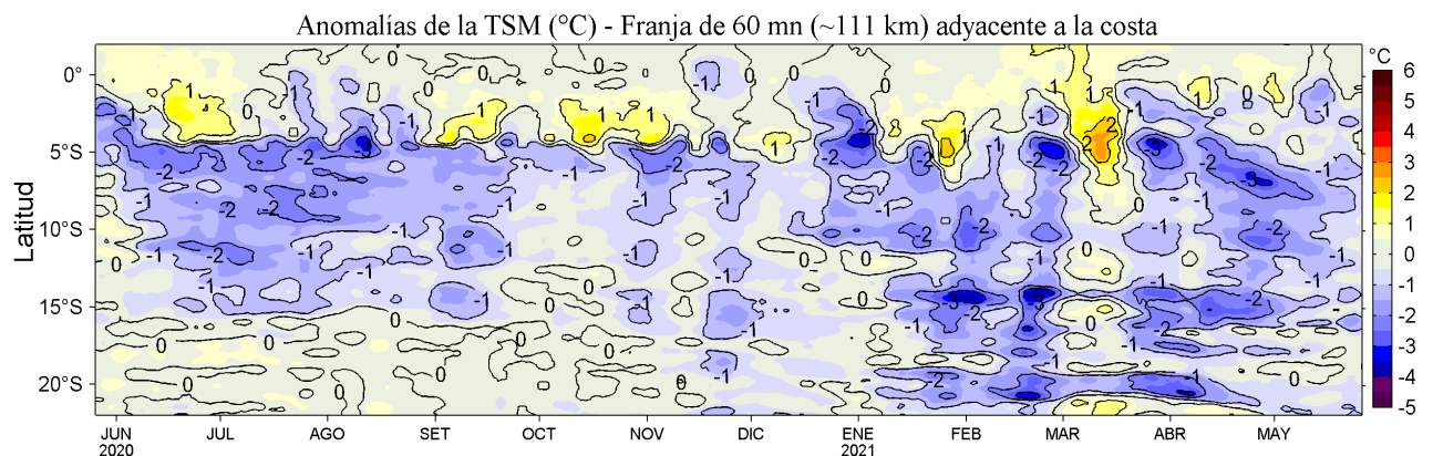
Figura 4. Variación promedio de las anomalías de la temperatura superficial del mar (TSM, °C) para una franja de 60 mn (~111 km) adyacente al litoral peruano para los últimos doce meses al 26 de mayo de 2021. Datos: OSTIA-UKMO-L4-GLOB-v2.0 (UK Met. Office, 2012; Donlon et al, 2012) disponible en https://podaac.jpl.nasa.gov/dataset/OSTIA-UKMO-L4-GLOB-v2.0 . Las anomalías se calcularon con respecto al periodo 2007-2016.
