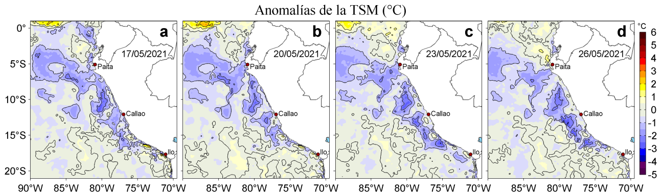
Figura 3. Anomalías de la temperatura superficial del mar (TSM, °C) para los días: a) 17, b) 20, c) 23 y d) 26 de mayo de 2021. Las anomalías se calcularon respecto de la climatología para el periodo 2007-2016. Datos: OSTIA-UKMO-L4-GLOB-v2.0 (UK Met Office, 2012; Donlon et al, 2012).
