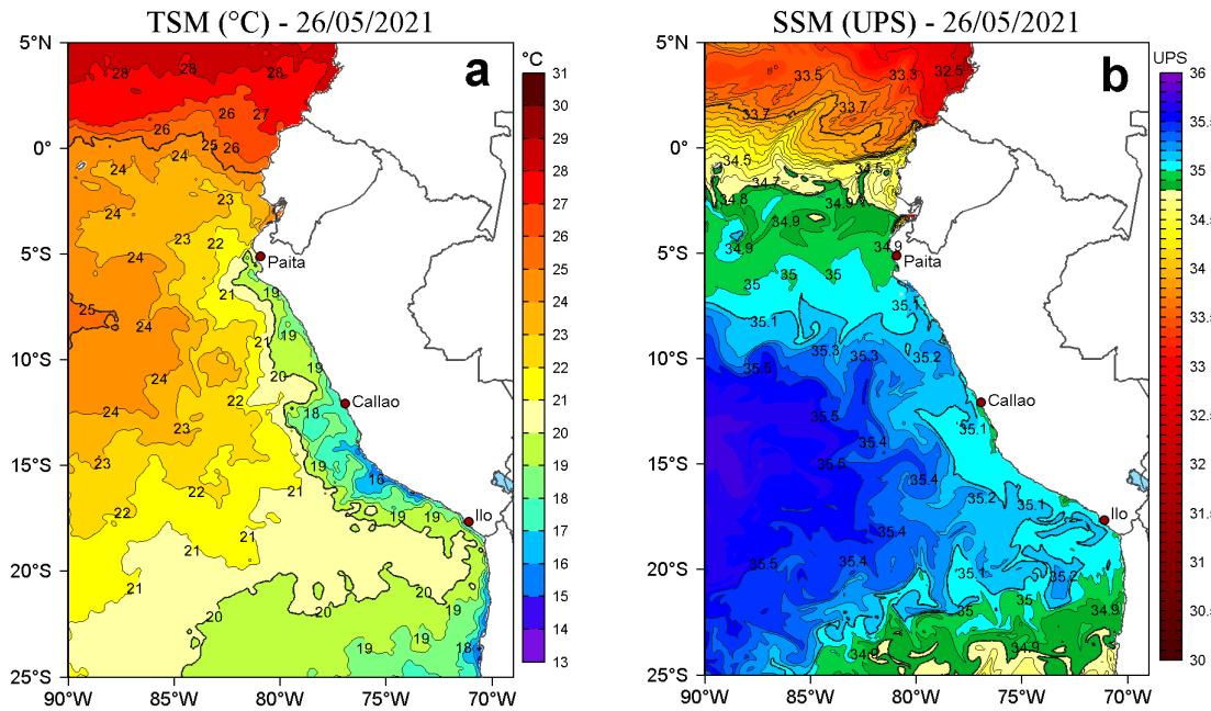
Figura 2. a) Temperatura superficial del mar (TSM, °C) y b) Salinidad superficial del mar (SSM) para el 26 de mayo de 2021. Datos: OSTIA-UKMO-L4-GLOB-v2.0 (UK Met Office, 2012; Donlon et al, 2012) disponible en https://podaac.jpl.nasa.gov/dataset/OSTIA-UKMO-L4-GLOB-v2.0 para (a) y Hybrid Coordinate Ocean Model v. GOFS 3.1 (HYCOM; Halliwell et al., 1998; 2000; Bleck, 2001) para (b).
