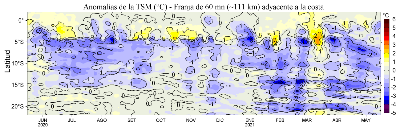
Figura 4. Variación promedio de las anomalías de la temperatura superficial del mar (TSM, °C) para una franja de 60 mn (~111 km) adyacente al litoral peruano para los últimos doce meses al 16 de mayo de 2021. Datos: OSTIA-UKMO-L4-GLOB-v2.0 (UK Met. Office, 2012; Donlon et al, 2012) disponible en https://podaac.jpl.nasa.gov/dataset/OSTIA-UKMO-L4-GLOB-v2.0 . Las anomalías se calcularon con respecto al periodo 2007-2016.
