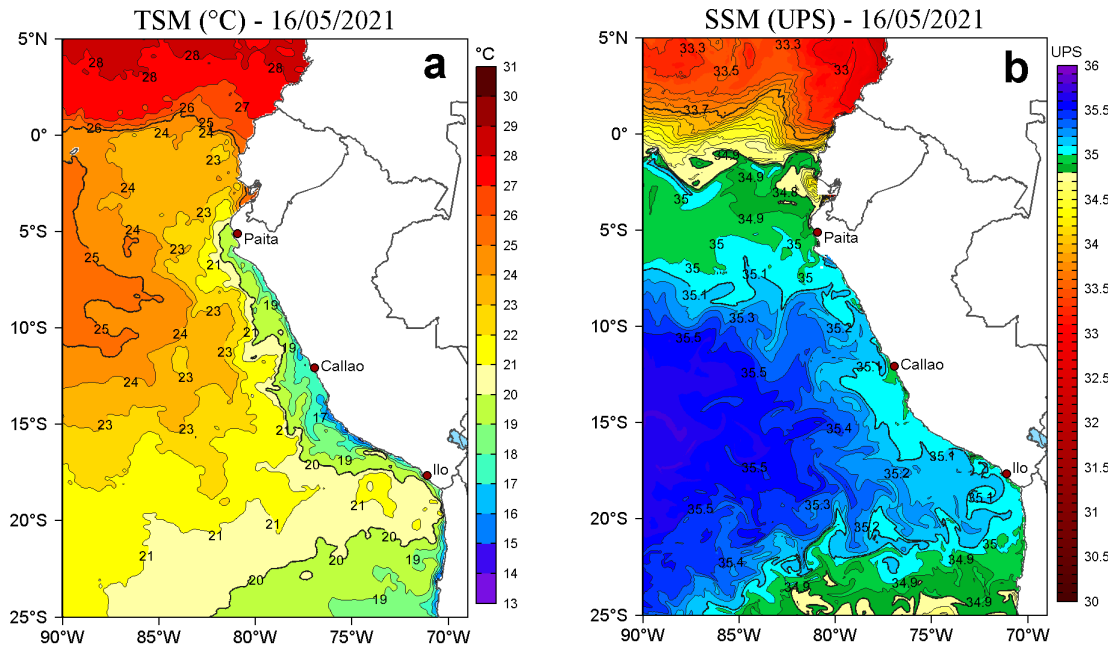
Figura 2. a) Temperatura superficial del mar (TSM, °C) y b) Salinidad superficial del mar (SSM) para el 16 de mayo de 2021. Datos: OSTIA-UKMO-L4-GLOB-v2.0 (UK Met Office, 2012; Donlon et al, 2012) disponible en https://podaac.jpl.nasa.gov/dataset/OSTIA-UKMO-L4-GLOB-v2.0 para (a) y Hybrid Coordinate Ocean Model v. GOFS 3.1 (HYCOM; Halliwell et al., 1998; 2000; Bleck, 2001) para (b).
