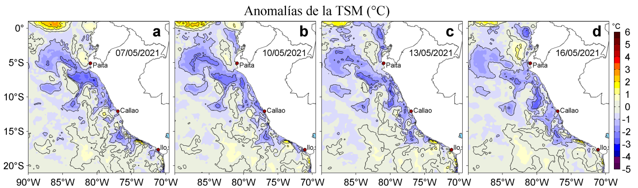
Figura 3. Anomalías de la temperatura superficial del mar (TSM, °C) para los días: a) 07, b) 10, c) 13 y d) 16 de mayo de 2021. Las anomalías se calcularon respecto de la climatología para el periodo 2007-2016. Datos: OSTIA-UKMO-L4-GLOB-v2.0 (UK Met Office, 2012; Donlon et al, 2012).
