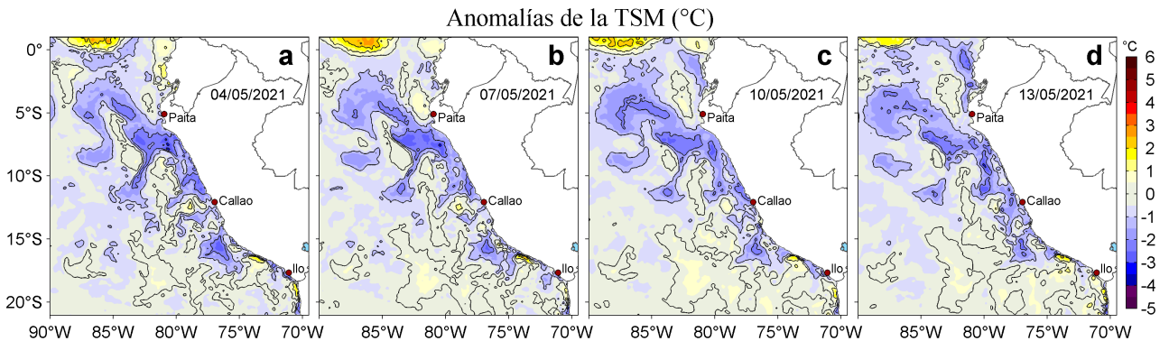
Figura 3. Anomalías de la temperatura superficial del mar (TSM, °C) para los días: a) 04, b) 07, c) 10 y d) 13 de mayo de 2021. Las anomalías se calcularon respecto de la climatología para el periodo 2007-2016. Datos: OSTIA-UKMO-L4-GLOB-v2.0 (UK Met Office, 2012; Donlon et al, 2012).
