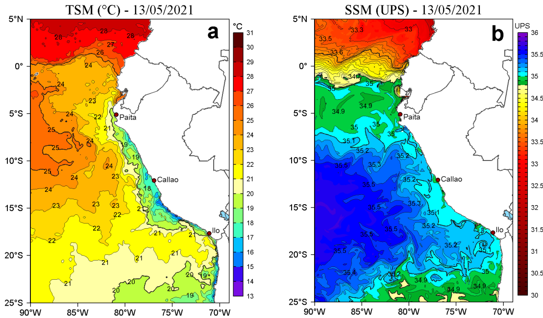
Figura 2. a) Temperatura superficial del mar (TSM, °C) y b) Salinidad superficial del mar (SSM) para el 13 de mayo de 2021. Datos: OSTIA-UKMO-L4-GLOB-v2.0 (UK Met Office, 2012; Donlon et al, 2012) disponible en https://podaac.jpl.nasa.gov/dataset/OSTIA-UKMO-L4-GLOB-v2.0 para (a) y Hybrid Coordinate Ocean Model v. GOFS 3.1 (HYCOM; Halliwell et al., 1998; 2000; Bleck, 2001) para (b).
