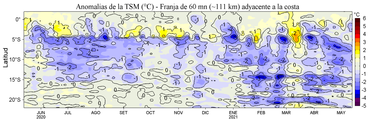
Figura 4. Variación promedio de las anomalías de la temperatura superficial del mar (TSM, °C) para una franja de 60 mn (~111 km) adyacente al litoral peruano para los últimos doce meses al 13 de mayo de 2021. Datos: OSTIA-UKMO-L4-GLOB-v2.0 (UK Met. Office, 2012; Donlon et al, 2012) disponible en https://podaac.jpl.nasa.gov/dataset/OSTIA-UKMO-L4-GLOB-v2.0 . Las anomalías se calcularon con respecto al periodo 2007-2016.
