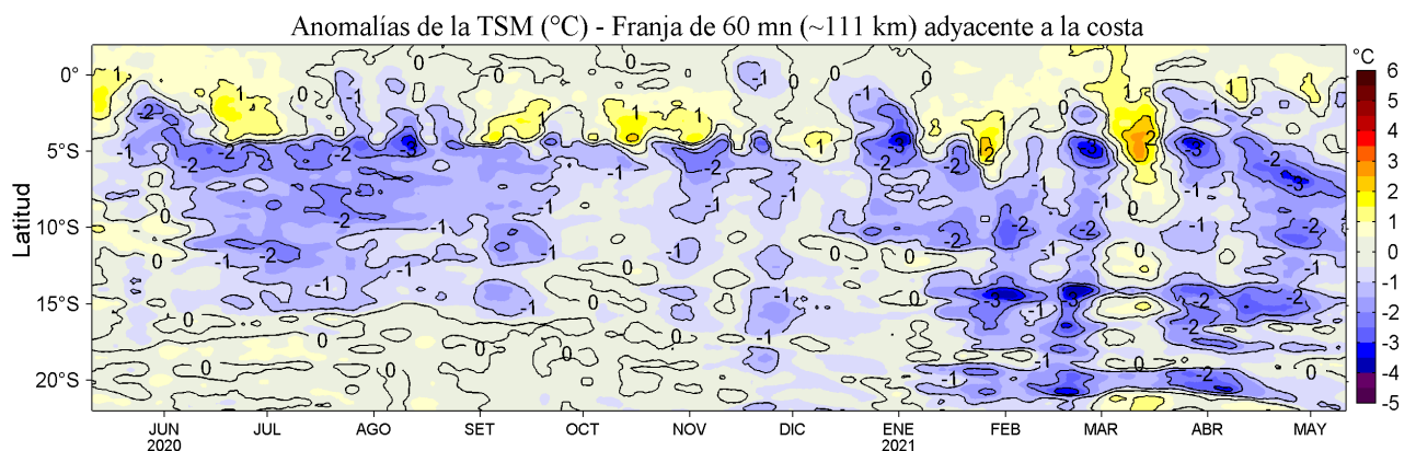
Figura 4. Variación promedio de las anomalías de la temperatura superficial del mar (TSM, °C) para una franja de 60 mn (~111 km) adyacente al litoral peruano para los últimos doce meses al 11 de mayo de 2021. Datos: OSTIA-UKMO-L4-GLOB-v2.0 (UK Met. Office, 2012; Donlon et al, 2012) disponible en https://podaac.jpl.nasa.gov/dataset/OSTIA-UKMO-L4-GLOB-v2.0 . Las anomalías se calcularon con respecto al periodo 2007-2016.
