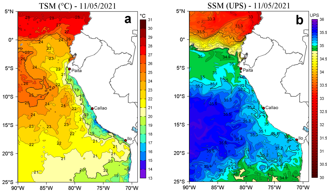
Figura 2. a) Temperatura superficial del mar (TSM, °C) y b) Salinidad superficial del mar (SSM) para el 11 de mayo de 2021. Datos: OSTIA-UKMO-L4-GLOB-v2.0 (UK Met Office, 2012; Donlon et al, 2012) disponible en https://podaac.jpl.nasa.gov/dataset/OSTIA-UKMO-L4-GLOB-v2.0 para (a) y Hybrid Coordinate Ocean Model v. GOF5 3.1 (HYCOM; Halliwell et al., 1998; 2000; Bleck, 2001) para (b).
