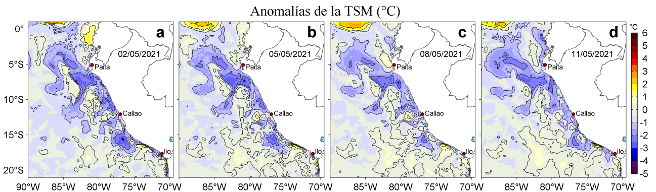
Figura 3. Anomalías de la temperatura superficial del mar (TSM, °C) para los días: a) 02, b) 05, c) 08 y d) 11 de mayo de 2021. Las anomalías se calcularon respecto de la climatología para el periodo 2007-2016. Datos: OSTIA-UKMO-L4-GLOB-v2.0 (UK Met Office, 2012; Donlon et al, 2012).
