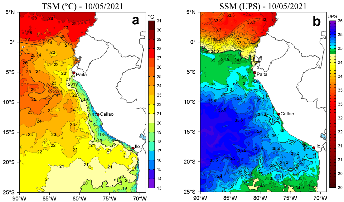
Figura 2. a) Temperatura superficial del mar (TSM, °C) y b) Salinidad superficial del mar (SSM) para el 10 de mayo de 2021. Datos: OSTIA-UKMO-L4-GLOB-v2.0 (UK Met Office, 2012; Donlon et al, 2012) disponible en https://podaac.jpl.nasa.gov/dataset/OSTIA-UKMO-L4-GLOB-v2.0 para (a) y Hybrid Coordinate Ocean Model v. GOFS 3.1 (HYCOM; Halliwell et al., 1998; 2000; Bleck, 2001) para (b).
