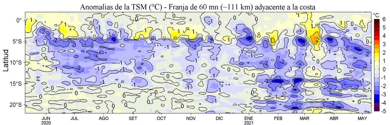
Figura 4. Variación promedio de las anomalías de la temperatura superficial del mar (TSM, °C) para una franja de 60 mn (~111 km) adyacente al litoral peruano para los últimos doce meses al 10 de mayo de 2021. Datos: OSTIA-UKMO-L4-GLOB-v2.0 (UK Met. Office, 2012; Donlon et al, 2012) disponible en https://podaac.jpl.nasa.gov/dataset/OSTIA-UKMO-L4-GLOB-v2.0 . Las anomalías se calcularon con respecto al periodo 2007-2016.
