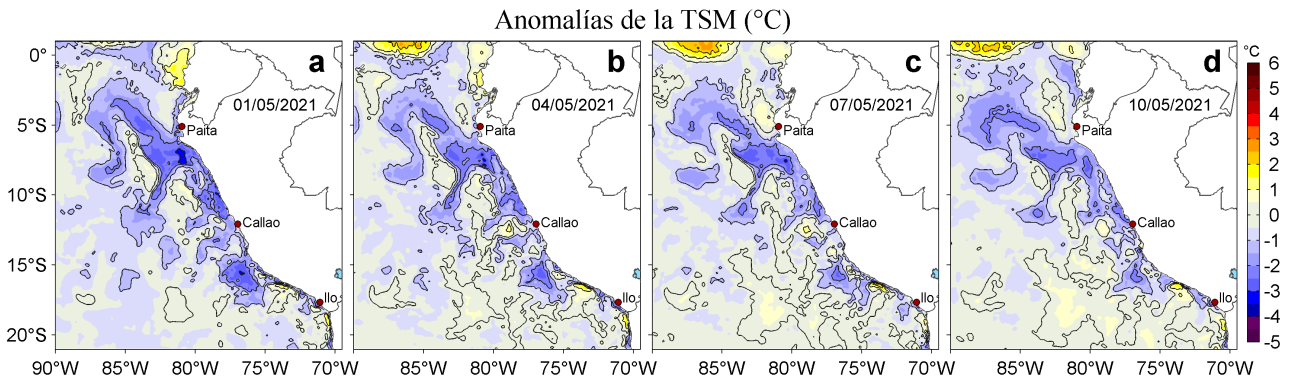
Figura 3. Anomalías de la temperatura superficial del mar (TSM, °C) para los días: a) 01, b) 04, c) 07 y d) 10 de mayo de 2021. Las anomalías se calcularon respecto de la climatología para el periodo 2007-2016. Datos: OSTIA-UKMO-L4-GLOB-v2.0 (UK Met Office, 2012; Donlon et al, 2012).
