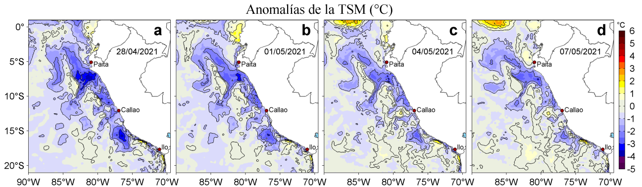
Figura 3. Anomalías de la temperatura superficial del mar (TSM, °C) para los días: a) 28 de abril, b) 01, c) 04 y d) 07 de mayo de 2021. Las anomalías se calcularon respecto de la climatología para el periodo 2007-2016. Datos: OSTIA-UKMO-L4-GLOB-v2.0 (UK Met Office, 2012; Donlon et al, 2012).
