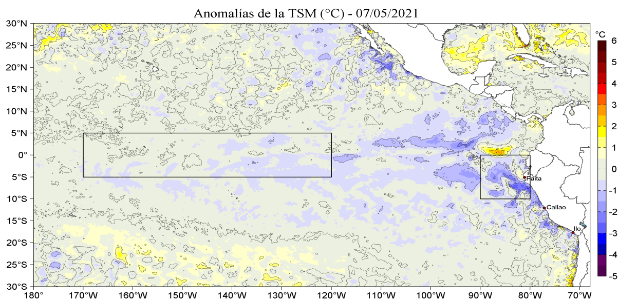
Figura 1. Anomalías de la temperatura superficial del mar (TSM, ^{\circ}\text{C} ) en el océano Pacífico tropical. Las regiones Niño 3.4 ( 5\text{ }^{\circ}\text{N} - 5\text{ }^{\circ}\text{S} , 170\text{ }^{\circ}\text{W} - 120\text{ }^{\circ}\text{W} ) y Niño 1+2 ( 0\text{ }^{\circ} - 10\text{ }^{\circ}\text{S} , 90\text{ }^{\circ}\text{W} - 80\text{ }^{\circ}\text{W} ) en los sectores central y oriental del océano, respectivamente, están delimitadas con una línea de color negro. Las anomalías se estimaron de acuerdo a la climatología para el periodo 2007-2016. Los datos provienen de OSTIA-UKMO-L4-GLOB-v2.0 (UK Met Office, 2012; Donlon et al, 2012) y están disponibles en https://podaac.jpl.nasa.gov/dataset/OSTIA-UKMO-L4-GLOB-v2.0 .
