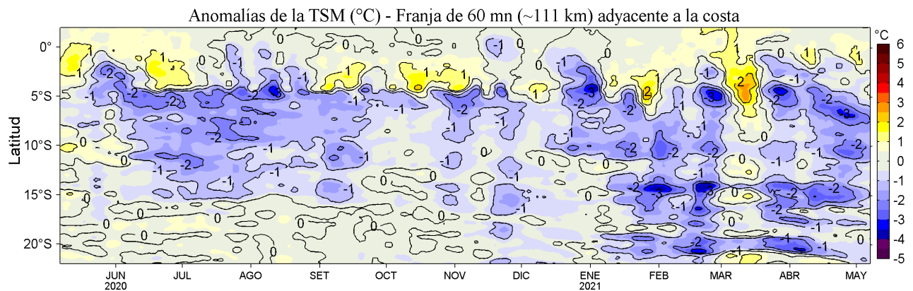
Figura 4. Variación promedio de las anomalías de la temperatura superficial del mar (TSM, °C) para una franja de 60 mn (~111 km) adyacente al litoral peruano para los últimos doce meses al 07 de mayo de 2021. Datos: OSTIA-UKMO-L4-GLOB-v2.0 (UK Met. Office, 2012; Donlon et al, 2012) disponible en https://podaac.jpl.nasa.gov/dataset/OSTIA-UKMO-L4-GLOB-v2.0 . Las anomalías se calcularon con respecto al periodo 2007-2016.
