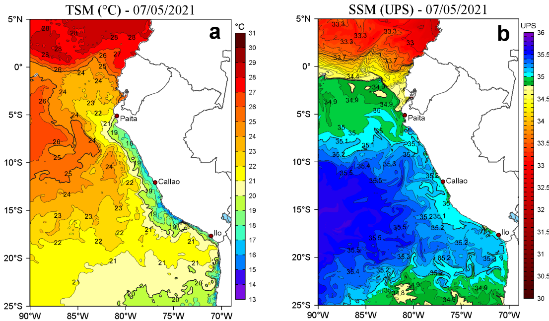
Figura 2. a) Temperatura superficial del mar (TSM, °C) y b) Salinidad superficial del mar (SSM) para el 07 de mayo de 2021. Datos: OSTIA-UKMO-L4-GLOB-v2.0 (UK Met Office, 2012; Donlon et al, 2012) disponible en https://podaac.jpl.nasa.gov/dataset/OSTIA-UKMO-L4-GLOB-v2.0 para (a) y Hybrid Coordinate Ocean Model v. GOF5 3.1 (HYCOM; Halliwell et al., 1998; 2000; Bleck, 2001) para (b).
