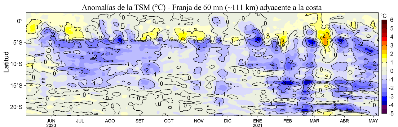
Figura 4. Variación promedio de las anomalías de la temperatura superficial del mar (TSM, °C) para una franja de 60 mn (~111 km) adyacente al litoral peruano para los últimos doce meses al 06 de mayo de 2021. Datos: OSTIA-UKMO-L4-GLOB-v2.0 (UK Met. Office, 2012; Donlon et al, 2012) disponible en https://podaac.jpl.nasa.gov/dataset/OSTIA-UKMO-L4-GLOB-v2.0 . Las anomalías se calcularon con respecto al periodo 2007-2016.
