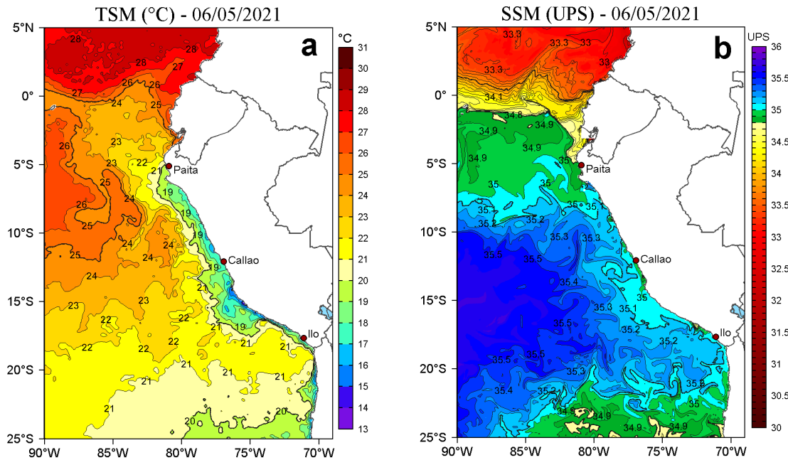
Figura 2. a) Temperatura superficial del mar (TSM, °C) y b) Salinidad superficial del mar (SSM) para el 06 de mayo de 2021. Datos: OSTIA-UKMO-L4-GLOB-v2.0 (UK Met Office, 2012; Donlon et al, 2012) disponible en https://podaac.jpl.nasa.gov/dataset/OSTIA-UKMO-L4-GLOB-v2.0 para (a) y Hybrid Coordinate Ocean Model v. GOFS 3.1 (HYCOM; Halliwell et al., 1998; 2000; Bleck, 2001) para (b).
