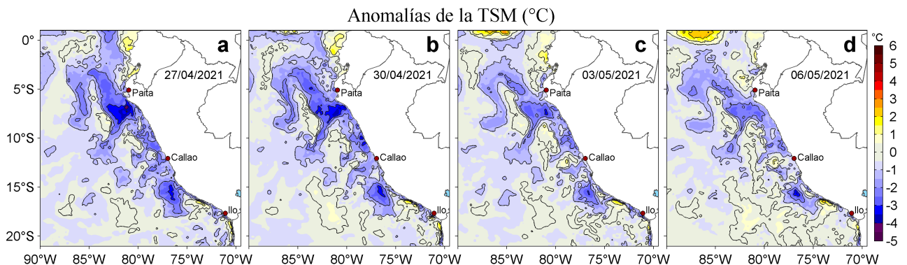
Figura 3. Anomalías de la temperatura superficial del mar (TSM, °C) para los días: a) 27 y b) 30 de abril, c) 03 y d) 06 de mayo de 2021. Las anomalías se calcularon respecto de la climatología para el periodo 2007-2016. Datos: OSTIA-UKMO-L4-GLOB-v2.0 (UK Met Office, 2012; Donlon et al, 2012).
