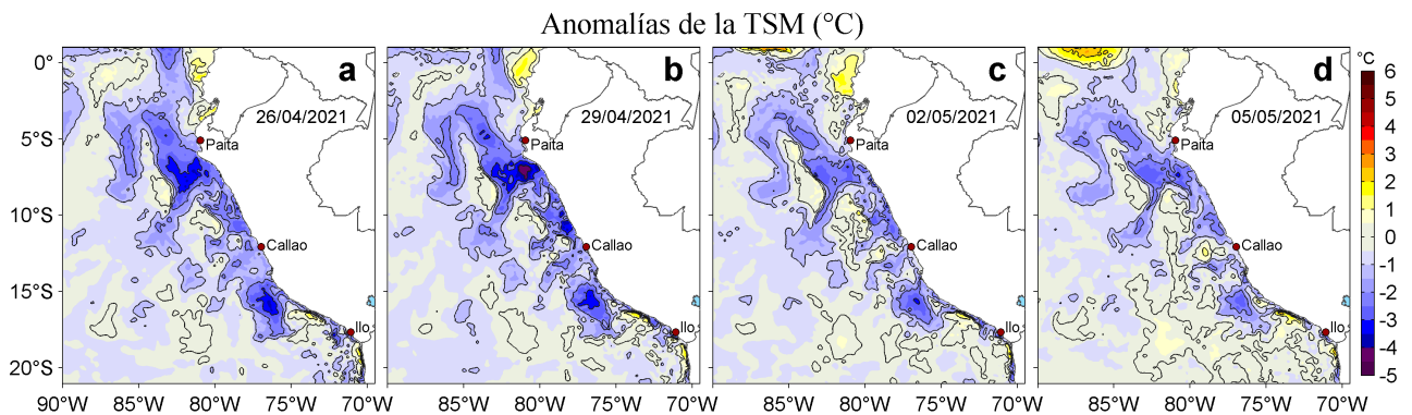
Figura 3. Anomalías de la temperatura superficial del mar (TSM, °C) para los días: a) 26 y b) 29 de abril, c) 02 y d) 05 de mayo de 2021. Las anomalías se calcularon respecto de la climatología para el periodo 2007-2016. Datos: OSTIA-UKMO-L4-GLOB-v2.0 (UK Met Office, 2012; Donlon et al, 2012).
