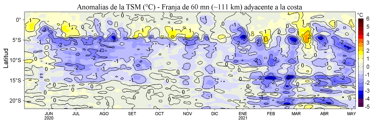
Figura 4. Variación promedio de las anomalías de la temperatura superficial del mar (TSM, °C) para una franja de 60 mn (~111 km) adyacente al litoral peruano para los últimos doce meses al 05 de mayo de 2021. Datos: OSTIA-UKMO-L4-GLOB-v2.0 (UK Met. Office, 2012; Donlon et al, 2012) disponible en https://podaac.jpl.nasa.gov/dataset/OSTIA-UKMO-L4-GLOB-v2.0 . Las anomalías se calcularon con respecto al periodo 2007-2016.
