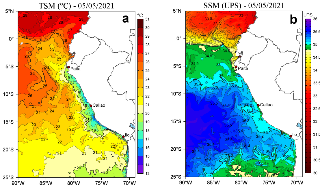
Figura 2. a) Temperatura superficial del mar (TSM, °C) y b) Salinidad superficial del mar (SSM) para el 05 de mayo de 2021. Datos: OSTIA-UKMO-L4-GLOB-v2.0 (UK Met Office, 2012; Donlon et al, 2012) disponible en https://podaac.jpl.nasa.gov/dataset/OSTIA-UKMO-L4-GLOB-v2.0 para (a) y Hybrid Coordinate Ocean Model v. GOFS 3.1 (HYCOM; Halliwell et al., 1998; 2000; Bleck, 2001) para (b).
