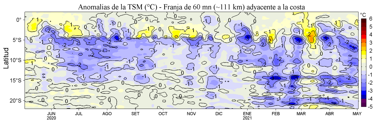
Figura 4. Variación promedio de las anomalías de la temperatura superficial del mar (TSM, °C) para una franja de 60 mn (~111 km) adyacente al litoral peruano para los últimos doce meses al 02 de mayo de 2021. Datos: OSTIA-UKMO-L4-GLOB-v2.0 (UK Met. Office, 2012; Donlon et al, 2012) disponible en https://podaac.jpl.nasa.gov/dataset/OSTIA-UKMO-L4-GLOB-v2.0 . Las anomalías se calcularon con respecto al periodo 2007-2016.
