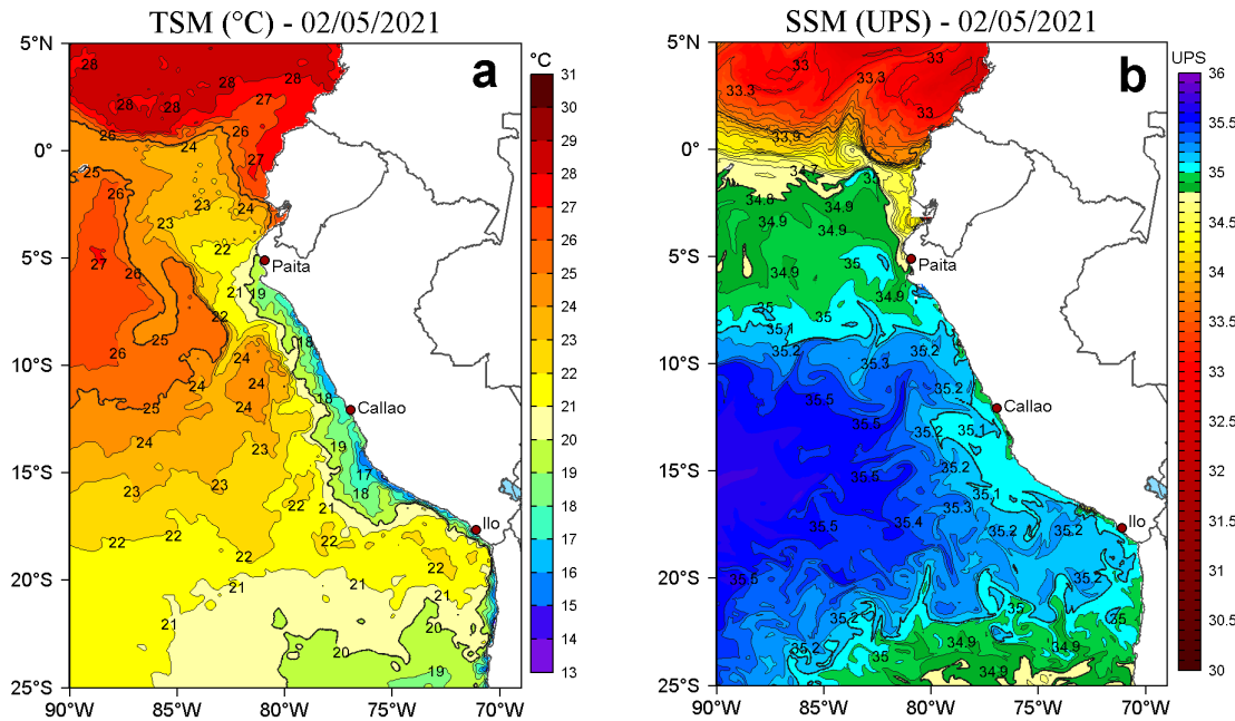
Figura 2. a) Temperatura superficial del mar (TSM, °C) y b) Salinidad superficial del mar (SSM) para el 02 de mayo de 2021. Datos: OSTIA-UKMO-L4-GLOB-v2.0 (UK Met Office, 2012; Donlon et al, 2012) disponible en https://podaac.jpl.nasa.gov/dataset/OSTIA-UKMO-L4-GLOB-v2.0 para (a) y Hybrid Coordinate Ocean Model v. GOF5 3.1 (HYCOM; Halliwell et al., 1998; 2000; Bleck, 2001) para (b).
