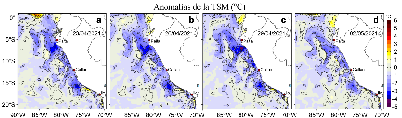
Figura 3. Anomalías de la temperatura superficial del mar (TSM, °C) para los días: a) 23, b) 26 y c) 29 de abril y d) 02 de mayo de 2021. Las anomalías se calcularon respecto de la climatología para el periodo 2007-2016. Datos: OSTIA-UKMO-L4-GLOB-v2.0 (UK Met Office, 2012; Donlon et al, 2012).
