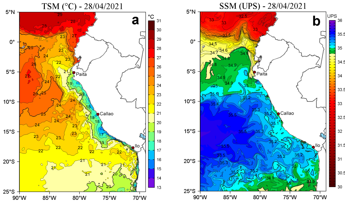
Figura 2. a) Temperatura superficial del mar (TSM, °C) y b) Salinidad superficial del mar (SSM) para el 28 de abril de 2021. Datos: OSTIA-UKMO-L4-GLOB-v2.0 (UK Met Office, 2012; Donlon et al, 2012) disponible en https://podaac.jpl.nasa.gov/dataset/OSTIA-UKMO-L4-GLOB-v2.0 para (a) y Hybrid Coordinate Ocean Model v. GOF5 3.1 (HYCOM; Halliwell et al., 1998; 2000; Bleck, 2001) para (b).
