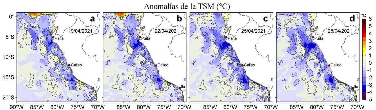
Figura 3. Anomalías de la temperatura superficial del mar (TSM, °C) para los días: a) 19, b) 22, c) 25 y d) 28 de abril de 2021. Las anomalías se calcularon respecto de la climatología para el periodo 2007-2016. Datos: OSTIA-UKMO-L4-GLOB-v2.0 (UK Met Office, 2012; Donlon et al, 2012).
