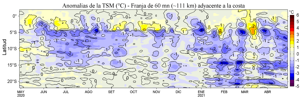
Figura 4. Variación promedio de las anomalías de la temperatura superficial del mar (TSM, °C) para una franja de 60 mn (~111 km) adyacente al litoral peruano para los últimos doce meses al 28 de abril de 2021. Datos: OSTIA-UKMO-L4-GLOB-v2.0 (UK Met. Office, 2012; Donlon et al, 2012) disponible en https://podaac.jpl.nasa.gov/dataset/OSTIA-UKMO-L4-GLOB-v2.0 . Las anomalías se calcularon con respecto al periodo 2007-2016.
