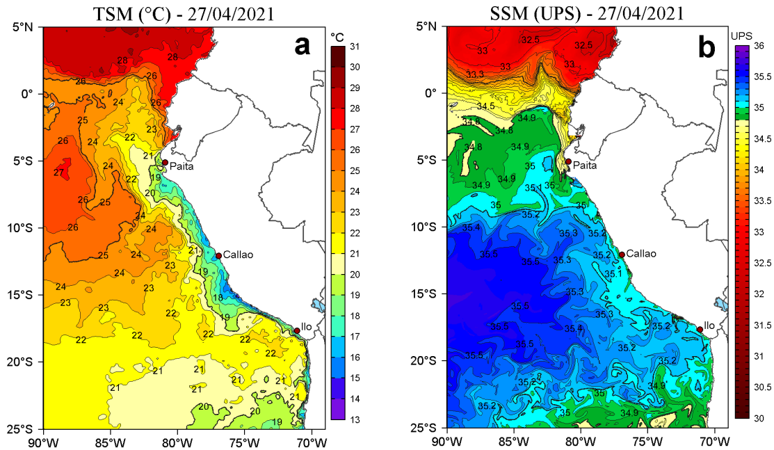
Figura 2. a) Temperatura superficial del mar (TSM, °C) y b) Salinidad superficial del mar (SSM) para el 27 de abril de 2021. Datos: OSTIA-UKMO-L4-GLOB-v2.0 (UK Met Office, 2012; Donlon et al, 2012) disponible en https://podaac.jpl.nasa.gov/dataset/OSTIA-UKMO-L4-GLOB-v2.0 para (a) y Hybrid Coordinate Ocean Model v. GOFS 3.1 (HYCOM; Halliwell et al., 1998; 2000; Bleck, 2001) para (b).
