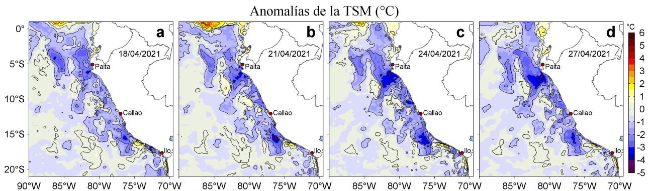
Figura 3. Anomalías de la temperatura superficial del mar (TSM, °C) para los días: a) 18, b) 21, c) 24 y d) 27 de abril de 2021. Las anomalías se calcularon respecto de la climatología para el periodo 2007-2016. Datos: OSTIA-UKMO-L4-GLOB-v2.0 (UK Met Office, 2012; Donlon et al, 2012).
