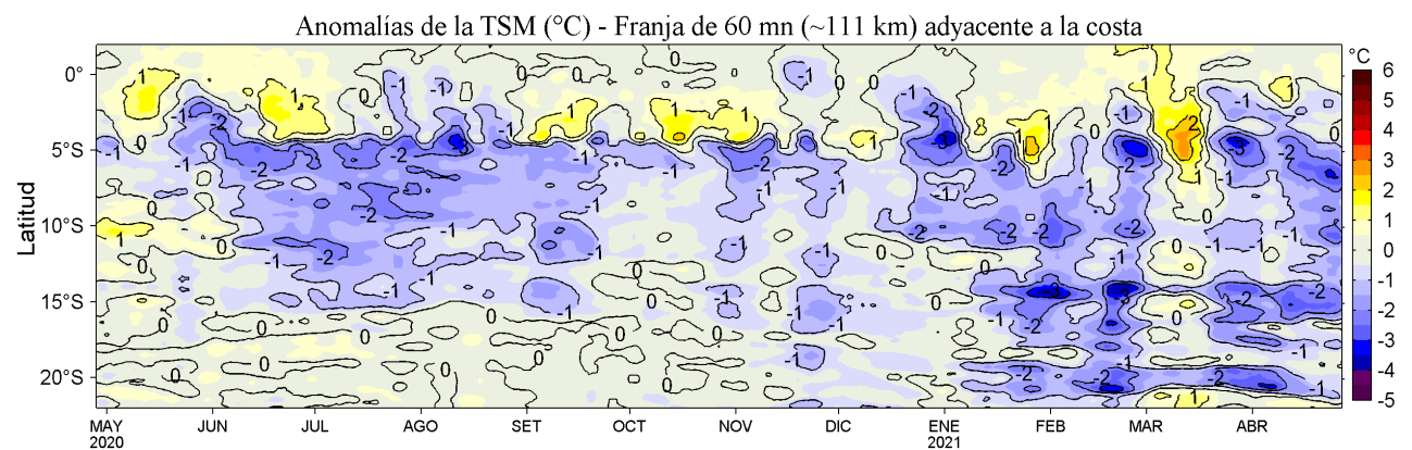
Figura 4. Variación promedio de las anomalías de la temperatura superficial del mar (TSM, °C) para una franja de 60 mn (~111 km) adyacente al litoral peruano para los últimos doce meses al 27 de abril de 2021. Datos: OSTIA-UKMO-L4-GLOB-v2.0 (UK Met. Office, 2012; Donlon et al, 2012) disponible en https://podaac.jpl.nasa.gov/dataset/OSTIA-UKMO-L4-GLOB-v2.0 . Las anomalías se calcularon con respecto al periodo 2007-2016.
