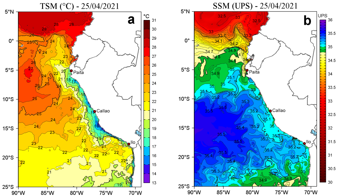
Figura 2. a) Temperatura superficial del mar (TSM, °C) y b) Salinidad superficial del mar (SSM) para el 25 de abril de 2021. Datos: OSTIA-UKMO-L4-GLOB-v2.0 (UK Met Office, 2012; Donlon et al, 2012) disponible en https://podaac.jpl.nasa.gov/dataset/OSTIA-UKMO-L4-GLOB-v2.0 para (a) y Hybrid Coordinate Ocean Model v. GOF5 3.1 (HYCOM; Halliwell et al., 1998; 2000; Bleck, 2001) para (b).
