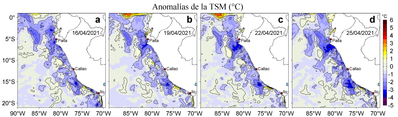
Figura 3. Anomalías de la temperatura superficial del mar (TSM, °C) para los días: a) 16, b) 19, c) 22 y d) 25 de abril de 2021. Las anomalías se calcularon respecto de la climatología para el periodo 2007-2016. Datos: OSTIA-UKMO-L4-GLOB-v2.0 (UK Met Office, 2012; Donlon et al, 2012).
