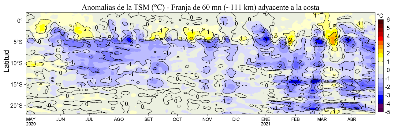
Figura 4. Variación promedio de las anomalías de la temperatura superficial del mar (TSM, °C) para una franja de 60 mn (~111 km) adyacente al litoral peruano para los últimos doce meses al 25 de abril de 2021. Datos: OSTIA-UKMO-L4-GLOB-v2.0 (UK Met. Office, 2012; Donlon et al, 2012) disponible en https://podaac.jpl.nasa.gov/dataset/OSTIA-UKMO-L4-GLOB-v2.0 . Las anomalías se calcularon con respecto al periodo 2007-2016.
