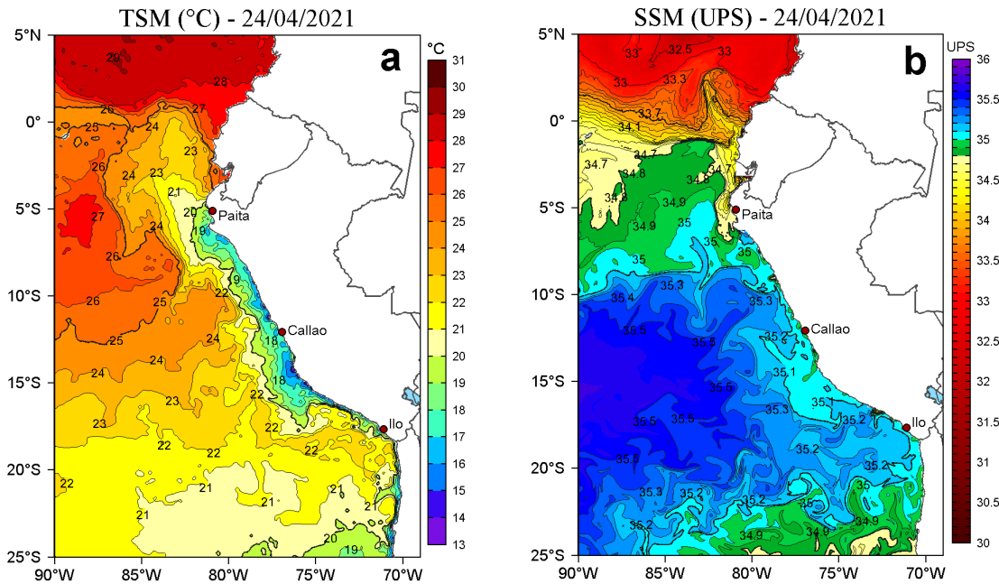
Figura 2. a) Temperatura superficial del mar (TSM, °C) y b) Salinidad superficial del mar (SSM) para el 24 de abril de 2021. Datos: OSTIA-UKMO-L4-GLOB-v2.0 (UK Met Office, 2012; Donlon et al, 2012) disponible en https://podaac.jpl.nasa.gov/dataset/OSTIA-UKMO-L4-GLOB-v2.0 para (a) y Hybrid Coordinate Ocean Model v. GOF5 3.1 (HYCOM; Halliwell et al., 1998; 2000; Bleck, 2001) para (b).
