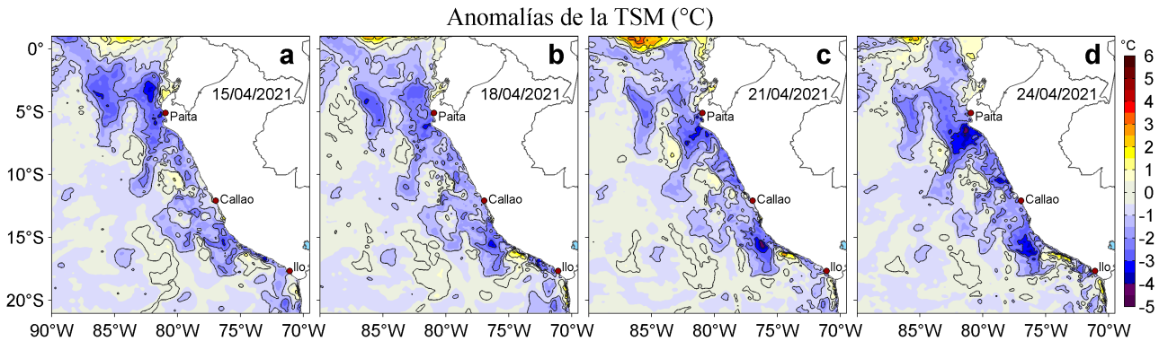
Figura 3. Anomalías de la temperatura superficial del mar (TSM, °C) para los días: a) 15, b) 18, c) 21 y d) 24 de abril de 2021. Las anomalías se calcularon respecto de la climatología para el periodo 2007-2016. Datos: OSTIA-UKMO-L4-GLOB-v2.0 (UK Met Office, 2012; Donlon et al, 2012).
