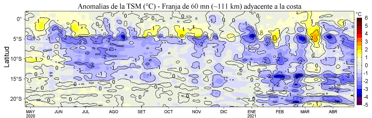
Figura 4. Variación promedio de las anomalías de la temperatura superficial del mar (TSM, °C) para una franja de 60 mn (~111 km) adyacente al litoral peruano para los últimos doce meses al 24 de abril de 2021. Datos: OSTIA-UKMO-L4-GLOB-v2.0 (UK Met. Office, 2012; Donlon et al, 2012) disponible en https://podaac.jpl.nasa.gov/dataset/OSTIA-UKMO-L4-GLOB-v2.0 . Las anomalías se calcularon con respecto al periodo 2007-2016.
