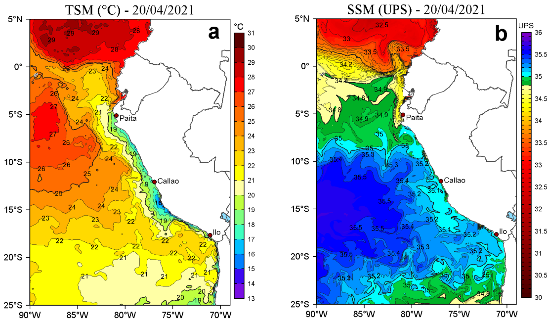
Figura 2. a) Temperatura superficial del mar (TSM, °C) y b) Salinidad superficial del mar (SSM) para el 20 de abril de 2021. Datos: OSTIA-UKMO-L4-GLOB-v2.0 (UK Met Office, 2012; Donlon et al, 2012) disponible en https://podaac.jpl.nasa.gov/dataset/OSTIA-UKMO-L4-GLOB-v2.0 para (a) y Hybrid Coordinate Ocean Model v. GOFS 3.1 (HYCOM; Halliwell et al., 1998; 2000; Bleck, 2001) para (b).
