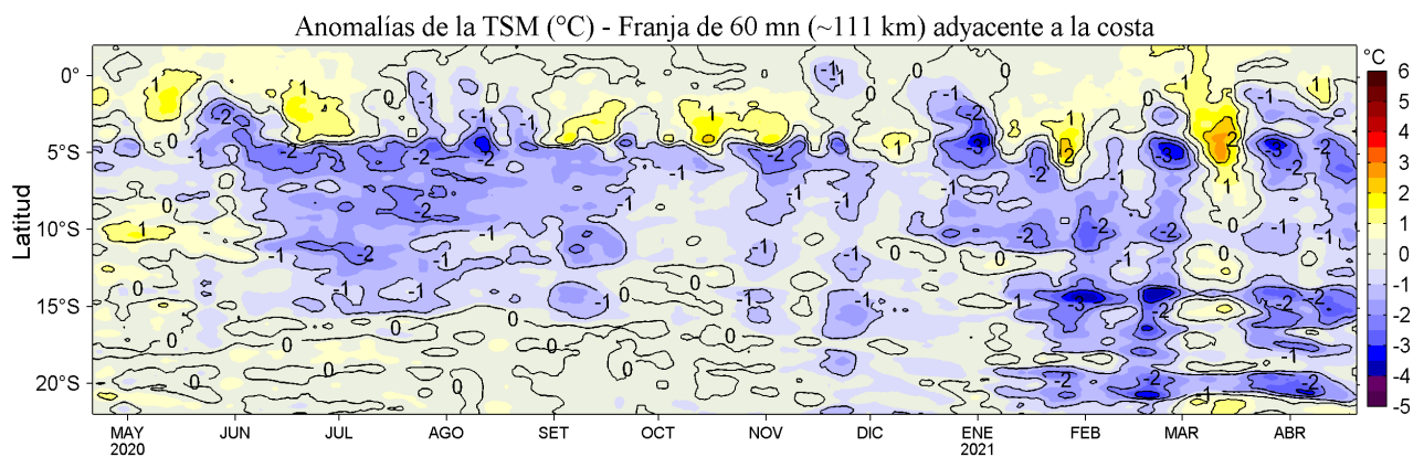
Figura 4. Variación promedio de las anomalías de la temperatura superficial del mar (TSM, °C) para una franja de 60 mn (~111 km) adyacente al litoral peruano para los últimos doce meses al 20 de abril de 2021. Datos: OSTIA-UKMO-L4-GLOB-v2.0 (UK Met. Office, 2012; Donlon et al, 2012) disponible en https://podaac.jpl.nasa.gov/dataset/OSTIA-UKMO-L4-GLOB-v2.0 . Las anomalías se calcularon con respecto al periodo 2007-2016.
