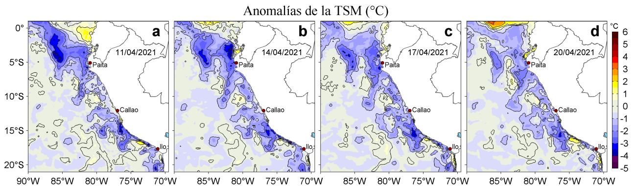
Figura 3. Anomalías de la temperatura superficial del mar (TSM, °C) para los días: a) 11, b) 14, c) 17 y d) 20 de abril de 2021. Las anomalías se calcularon respecto de la climatología para el periodo 2007-2016. Datos: OSTIA-UKMO-L4-GLOB-v2.0 (UK Met Office, 2012; Donlon et al, 2012).
