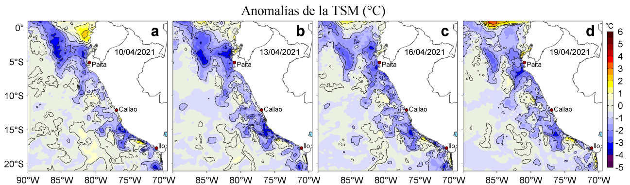
Figura 3. Anomalías de la temperatura superficial del mar (TSM, °C) para los días: a) 10, b) 13, c) 16 y d) 19 de abril de 2021. Las anomalías se calcularon respecto de la climatología para el periodo 2007-2016. Datos: OSTIA-UKMO-L4-GLOB-v2.0 (UK Met Office, 2012; Donlon et al, 2012).
