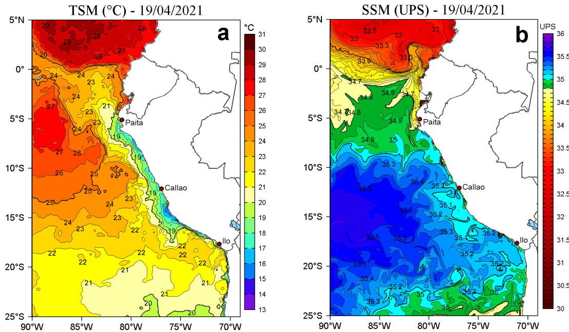
Figura 2. a) Temperatura superficial del mar (TSM, °C) y b) Salinidad superficial del mar (SSM) para el 19 de abril de 2021. Datos: OSTIA-UKMO-L4-GLOB-v2.0 (UK Met Office, 2012; Donlon et al, 2012) disponible en https://podaac.jpl.nasa.gov/dataset/OSTIA-UKMO-L4-GLOB-v2.0 para (a) y Hybrid Coordinate Ocean Model v. GOF5 3.1 (HYCOM; Halliwell et al., 1998; 2000; Bleck, 2001) para (b).
