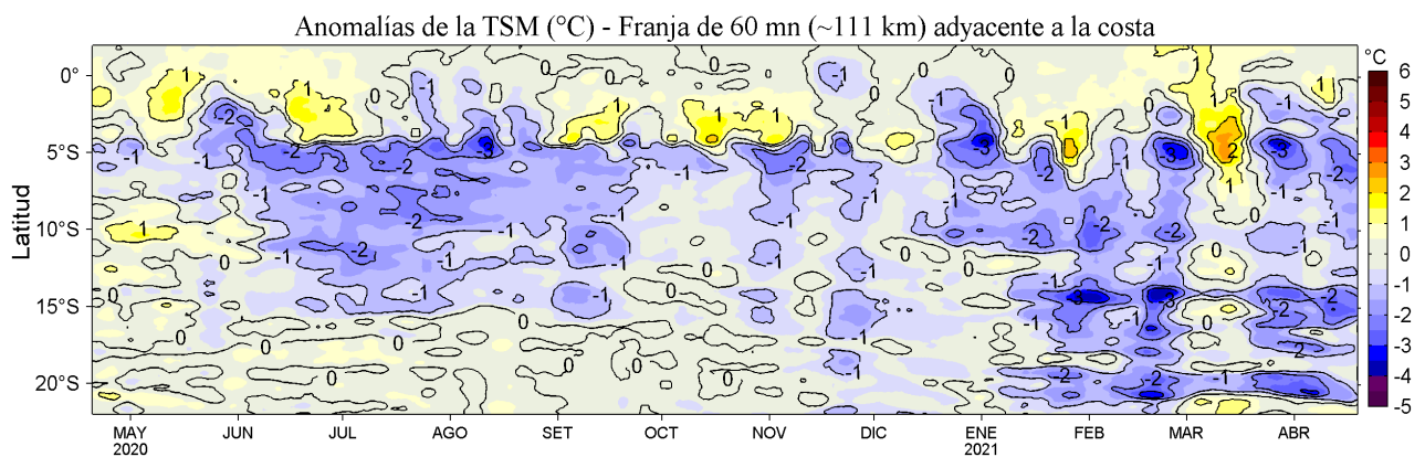
Figura 4. Variación promedio de las anomalías de la temperatura superficial del mar (TSM, °C) para una franja de 60 mn (~111 km) adyacente al litoral peruano para los últimos doce meses al 19 de abril de 2021. Datos: OSTIA-UKMO-L4-GLOB-v2.0 (UK Met. Office, 2012; Donlon et al, 2012) disponible en https://podaac.jpl.nasa.gov/dataset/OSTIA-UKMO-L4-GLOB-v2.0 . Las anomalías se calcularon con respecto al periodo 2007-2016.
