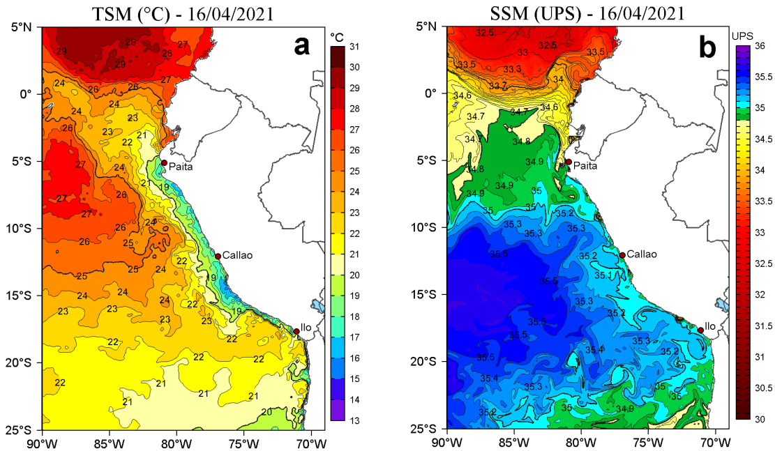
Figura 2. a) Temperatura superficial del mar (TSM, °C) y b) Salinidad superficial del mar (SSM) para el 16 de abril de 2021. Datos: OSTIA-UKMO-L4-GLOB-v2.0 (UK Met Office, 2012; Donlon et al, 2012) disponible en https://podaac.jpl.nasa.gov/dataset/OSTIA-UKMO-L4-GLOB-v2.0 para (a) y Hybrid Coordinate Ocean Model v. GOF5 3.1 (HYCOM; Halliwell et al., 1998; 2000; Bleck, 2001) para (b).
