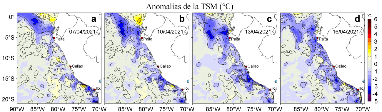
Figura 3. Anomalías de la temperatura superficial del mar (TSM, °C) para los días: a) 07, b) 10, c) 13 y d) 16 de abril de 2021. Las anomalías se calcularon respecto de la climatología para el periodo 2007-2016. Datos: OSTIA-UKMO-L4-GLOB-v2.0 (UK Met Office, 2012; Donlon et al, 2012).
