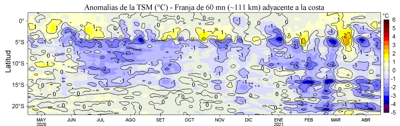
Figura 4. Variación promedio de las anomalías de la temperatura superficial del mar (TSM, °C) para una franja de 60 mn (~111 km) adyacente al litoral peruano para los últimos doce meses al 16 de abril de 2021. Datos: OSTIA-UKMO-L4-GLOB-v2.0 (UK Met. Office, 2012; Donlon et al, 2012) disponible en https://podaac.jpl.nasa.gov/dataset/OSTIA-UKMO-L4-GLOB-v2.0 . Las anomalías se calcularon con respecto al periodo 2007-2016.
