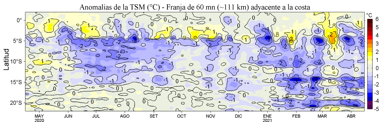
Figura 4. Variación promedio de las anomalías de la temperatura superficial del mar (TSM, °C) para una franja de 60 mn (~111 km) adyacente al litoral peruano para los últimos doce meses al 15 de abril de 2021. Datos: OSTIA-UKMO-L4-GLOB-v2.0 (UK Met. Office, 2012; Donlon et al, 2012) disponible en https://podaac.jpl.nasa.gov/dataset/OSTIA-UKMO-L4-GLOB-v2.0 . Las anomalías se calcularon con respecto al periodo 2007-2016.
