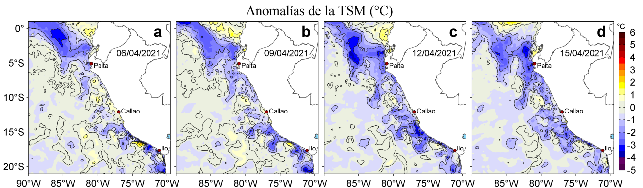
Figura 3. Anomalías de la temperatura superficial del mar (TSM, °C) para los días: a) 06, b) 09, c) 12 y d) 15 de abril de 2021. Las anomalías se calcularon respecto de la climatología para el periodo 2007-2016. Datos: OSTIA-UKMO-L4-GLOB-v2.0 (UK Met Office, 2012; Donlon et al, 2012).
