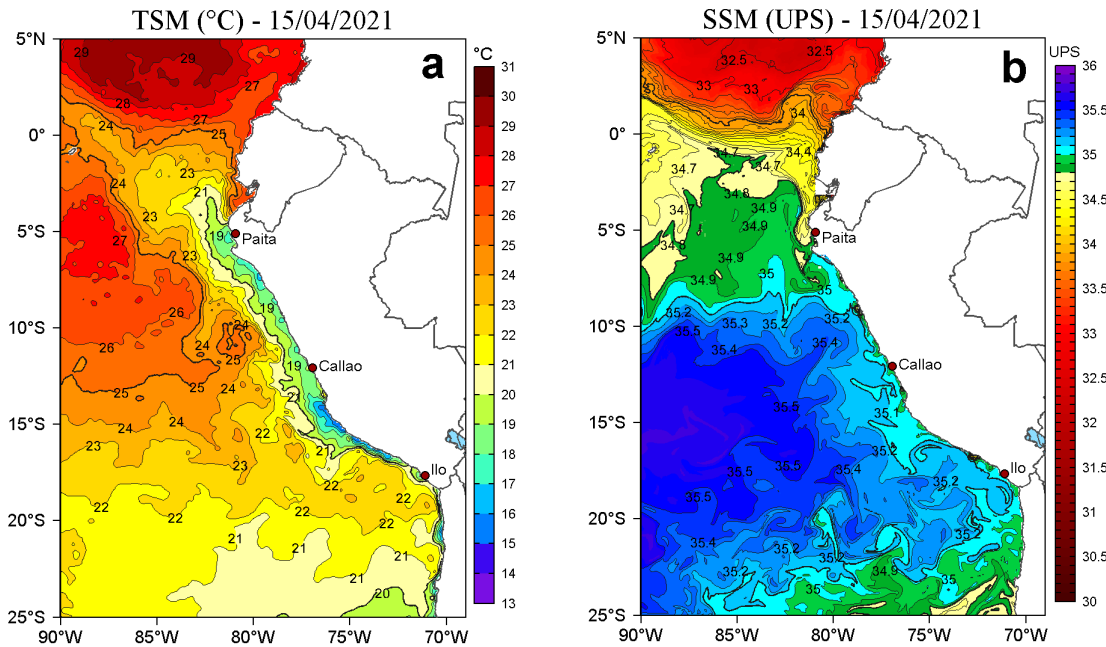
Figura 2. a) Temperatura superficial del mar (TSM, °C) y b) Salinidad superficial del mar (SSM) para el 15 de abril de 2021. Datos: OSTIA-UKMO-L4-GLOB-v2.0 (UK Met Office, 2012; Donlon et al, 2012) disponible en https://podaac.jpl.nasa.gov/dataset/OSTIA-UKMO-L4-GLOB-v2.0 para (a) y Hybrid Coordinate Ocean Model v. GOF5 3.1 (HYCOM; Halliwell et al., 1998; 2000; Bleck, 2001) para (b).
