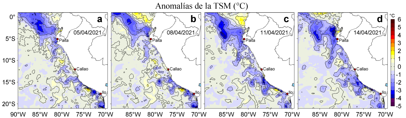
Figura 3. Anomalías de la temperatura superficial del mar (TSM, °C) para los días: a) 05, b) 08, c) 11 y d) 14 de abril de 2021. Las anomalías se calcularon respecto de la climatología para el periodo 2007-2016. Datos: OSTIA-UKMO-L4-GLOB-v2.0 (UK Met Office, 2012; Donlon et al, 2012).
