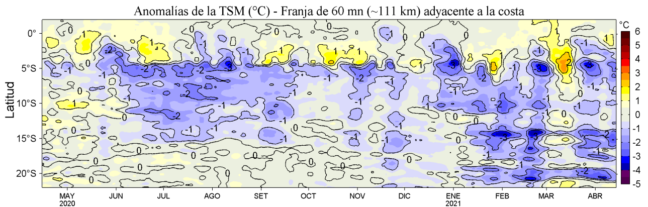
Figura 4. Variación promedio de las anomalías de la temperatura superficial del mar (TSM, °C) para una franja de 60 mn (~111 km) adyacente al litoral peruano para los últimos doce meses al 14 de abril de 2021. Datos: OSTIA-UKMO-L4-GLOB-v2.0 (UK Met. Office, 2012; Donlon et al, 2012) disponible en https://podaac.jpl.nasa.gov/dataset/OSTIA-UKMO-L4-GLOB-v2.0 . Las anomalías se calcularon con respecto al periodo 2007-2016.
