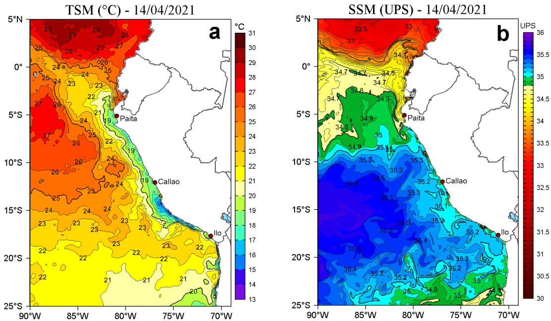
Figura 2. a) Temperatura superficial del mar (TSM, °C) y b) Salinidad superficial del mar (SSM) para el 14 de abril de 2021. Datos: OSTIA-UKMO-L4-GLOB-v2.0 (UK Met Office, 2012; Donlon et al, 2012) disponible en https://podaac.jpl.nasa.gov/dataset/OSTIA-UKMO-L4-GLOB-v2.0 para (a) y Hybrid Coordinate Ocean Model v. GOF5 3.1 (HYCOM; Halliwell et al., 1998; 2000; Bleck, 2001) para (b).
