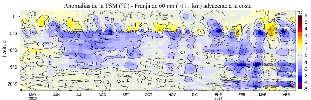
Figura 4. Variación promedio de las anomalías de la temperatura superficial del mar (TSM, °C) para una franja de 60 mn (~111 km) adyacente al litoral peruano para los últimos doce meses al 13 de abril de 2021. Datos: OSTIA-UKMO-L4-GLOB-v2.0 (UK Met. Office, 2012; Donlon et al, 2012) disponible en https://podaac.jpl.nasa.gov/dataset/OSTIA-UKMO-L4-GLOB-v2.0 . Las anomalías se calcularon con respecto al periodo 2007-2016.
