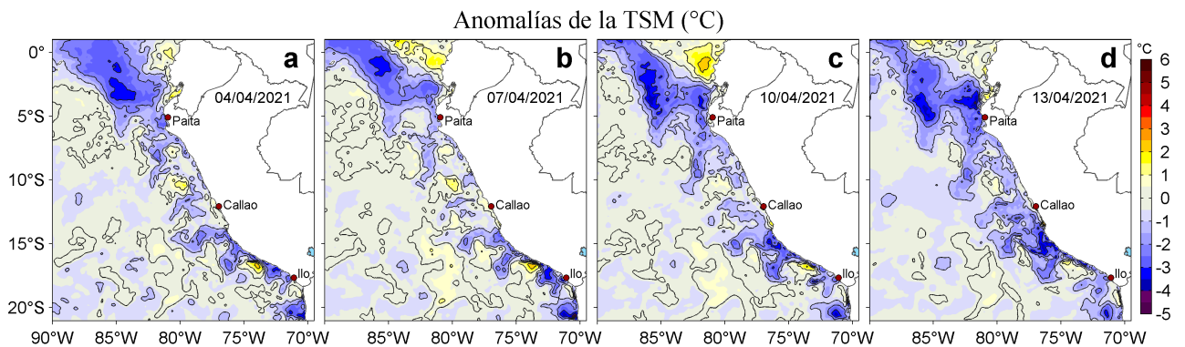
Figura 3. Anomalías de la temperatura superficial del mar (TSM, °C) para los días: a) 04, b) 07, c) 10 y d) 13 de abril de 2021. Las anomalías se calcularon respecto de la climatología para el periodo 2007-2016. Datos: OSTIA-UKMO-L4-GLOB-v2.0 (UK Met Office, 2012; Donlon et al, 2012).
