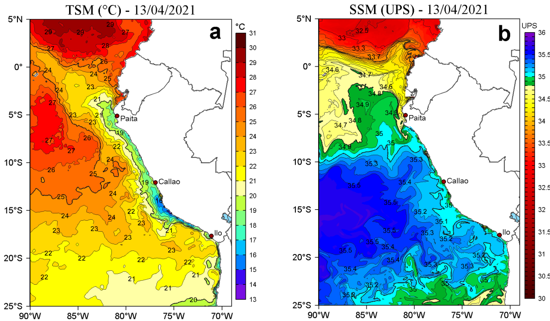
Figura 2. a) Temperatura superficial del mar (TSM, °C) y b) Salinidad superficial del mar (SSM) para el 13 de abril de 2021. Datos: OSTIA-UKMO-L4-GLOB-v2.0 (UK Met Office, 2012; Donlon et al, 2012) disponible en https://podaac.jpl.nasa.gov/dataset/OSTIA-UKMO-L4-GLOB-v2.0 para (a) y Hybrid Coordinate Ocean Model v. GOF5 3.1 (HYCOM; Halliwell et al., 1998; 2000; Bleck, 2001) para (b).
