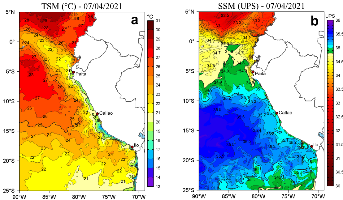
Figura 2. a) Temperatura superficial del mar (TSM, °C) y b) Salinidad superficial del mar (SSM) para el 07 de abril de 2021. Datos: OSTIA-UKMO-L4-GLOB-v2.0 (UK Met Office, 2012; Donlon et al, 2012) disponible en https://podaac.jpl.nasa.gov/dataset/OSTIA-UKMO-L4-GLOB-v2.0 para (a) y Hybrid Coordinate Ocean Model v. GOF5 3.1 (HYCOM; Halliwell et al., 1998; 2000; Bleck, 2001) para (b).
