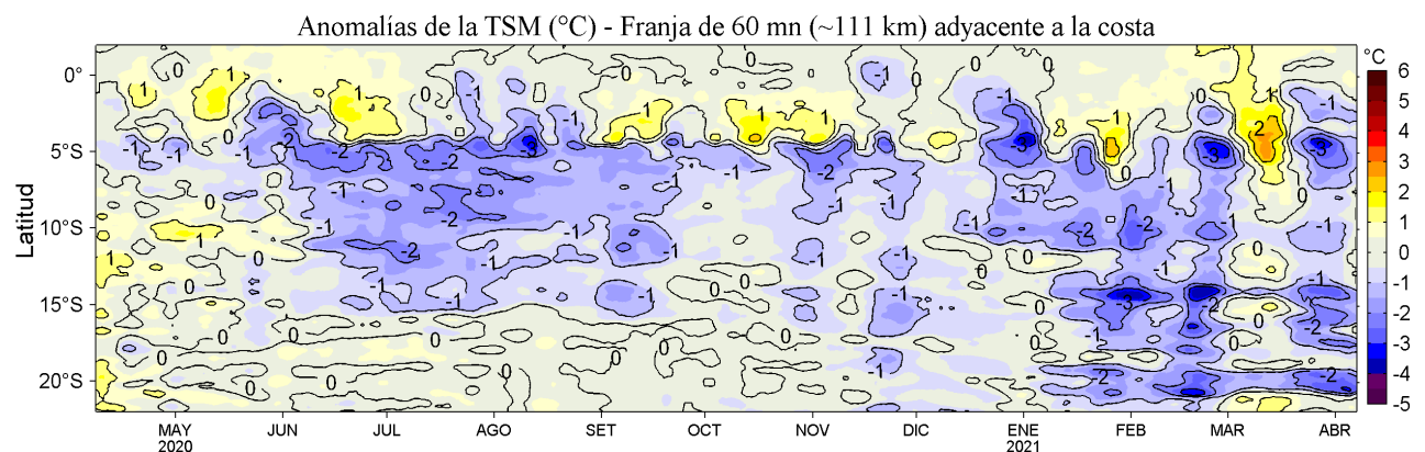
Figura 4. Variación promedio de las anomalías de la temperatura superficial del mar (TSM, °C) para una franja de 60 mn (~111 km) adyacente al litoral peruano para los últimos doce meses al 07 de abril de 2021. Datos: OSTIA-UKMO-L4-GLOB-v2.0 (UK Met. Office, 2012; Donlon et al, 2012) disponible en https://podaac.jpl.nasa.gov/dataset/OSTIA-UKMO-L4-GLOB-v2.0 . Las anomalías se calcularon con respecto al periodo 2007-2016.
