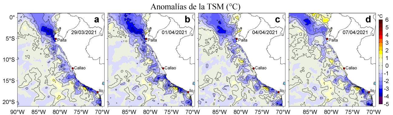
Figura 3. Anomalías de la temperatura superficial del mar (TSM, °C) para los días: a) 29 de marzo, b) 01, c) 04 y d) 07 de abril de 2021. Las anomalías se calcularon respecto de la climatología para el periodo 2007-2016. Datos: OSTIA-UKMO-L4-GLOB-v2.0 (UK Met Office, 2012; Donlon et al, 2012).
