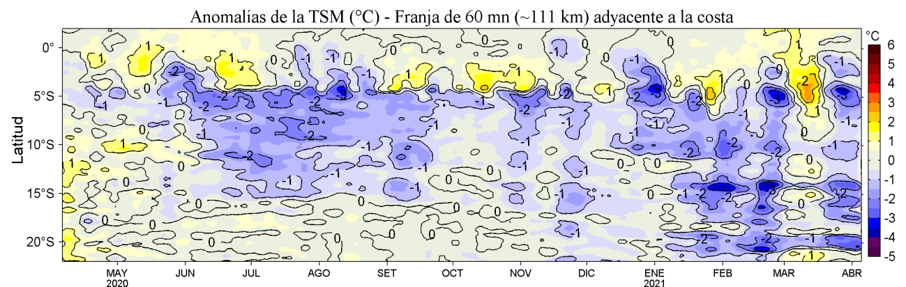
Figura 4. Variación promedio de las anomalías de la temperatura superficial del mar (TSM, °C) para una franja de 60 mn (~111 km) adyacente al litoral peruano para los últimos doce meses al 05 de abril de 2021. Datos: OSTIA-UKMO-L4-GLOB-v2.0 (UK Met. Office, 2012; Donlon et al, 2012) disponible en https://podaac.jpl.nasa.gov/dataset/OSTIA-UKMO-L4-GLOB-v2.0 . Las anomalías se calcularon con respecto al periodo 2007-2016.
