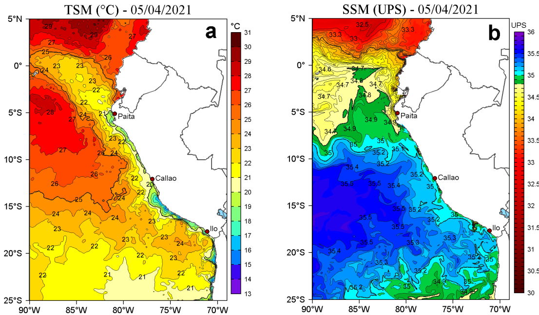
Figura 2. a) Temperatura superficial del mar (TSM, °C) y b) Salinidad superficial del mar (SSM) para el 05 de abril de 2021. Datos: OSTIA-UKMO-L4-GLOB-v2.0 (UK Met Office, 2012; Donlon et al, 2012) disponible en https://podaac.jpl.nasa.gov/dataset/OSTIA-UKMO-L4-GLOB-v2.0 para (a) y Hybrid Coordinate Ocean Model v. GOFS 3.1 (HYCOM; Halliwell et al., 1998; 2000; Bleck, 2001) para (b).
