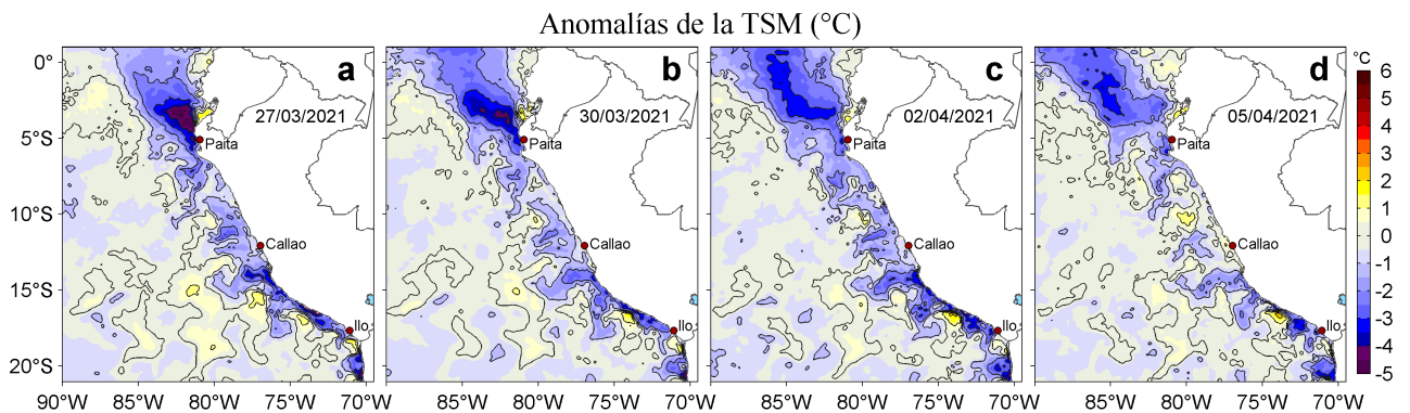
Figura 3. Anomalías de la temperatura superficial del mar (TSM, °C) para los días: a) 27 y b) 30 de marzo, c) 02 y d) 05 de abril de 2021. Las anomalías se calcularon respecto de la climatología para el periodo 2007-2016. Datos: OSTIA-UKMO-L4-GLOB-v2.0 (UK Met Office, 2012; Donlon et al, 2012).
