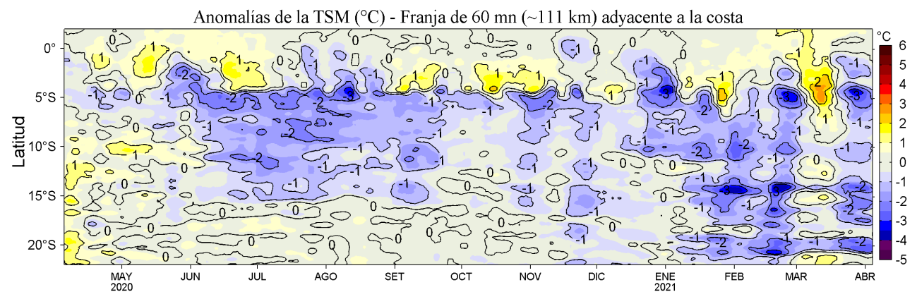
Figura 4. Variación promedio de las anomalías de la temperatura superficial del mar (TSM, °C) para una franja de 60 mn (~111 km) adyacente al litoral peruano para los últimos doce meses al 04 de abril de 2021. Datos: OSTIA-UKMO-L4-GLOB-v2.0 (UK Met. Office, 2012; Donlon et al, 2012) disponible en https://podaac.jpl.nasa.gov/dataset/OSTIA-UKMO-L4-GLOB-v2.0 . Las anomalías se calcularon con respecto al periodo 2007-2016.
