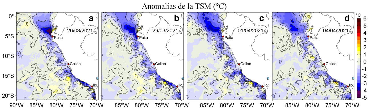
Figura 3. Anomalías de la temperatura superficial del mar (TSM, °C) para los días: a) 26 y b) 29 de marzo, c) 01 y d) 04 de abril de 2021. Las anomalías se calcularon respecto de la climatología para el periodo 2007-2016. Datos: OSTIA-UKMO-L4-GLOB-v2.0 (UK Met Office, 2012; Donlon et al, 2012).
