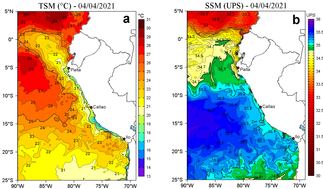
Figura 2. a) Temperatura superficial del mar (TSM, °C) y b) Salinidad superficial del mar (SSM) para el 04 de abril de 2021. Datos: OSTIA-UKMO-L4-GLOB-v2.0 (UK Met Office, 2012; Donlon et al, 2012) disponible en https://podaac.jpl.nasa.gov/dataset/OSTIA-UKMO-L4-GLOB-v2.0 para (a) y Hybrid Coordinate Ocean Model v. GOF5 3.1 (HYCOM; Halliwell et al., 1998; 2000; Bleck, 2001) para (b).
