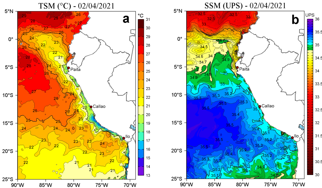
Figura 2. a) Temperatura superficial del mar (TSM, °C) y b) Salinidad superficial del mar (SSM) para el 02 de abril de 2021. Datos: OSTIA-UKMO-L4-GLOB-v2.0 (UK Met Office, 2012; Donlon et al, 2012) disponible en https://podaac.jpl.nasa.gov/dataset/OSTIA-UKMO-L4-GLOB-v2.0 para (a) y Hybrid Coordinate Ocean Model v. GOF5 3.1 (HYCOM; Halliwell et al., 1998; 2000; Bleck, 2001) para (b).
