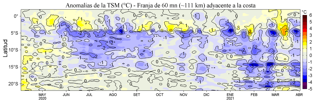
Figura 4. Variación promedio de las anomalías de la temperatura superficial del mar (TSM, °C) para una franja de 60 mn (~111 km) adyacente al litoral peruano para los últimos doce meses al 02 de abril de 2021. Datos: OSTIA-UKMO-L4-GLOB-v2.0 (UK Met. Office, 2012; Donlon et al, 2012) disponible en https://podaac.jpl.nasa.gov/dataset/OSTIA-UKMO-L4-GLOB-v2.0 . Las anomalías se calcularon con respecto al periodo 2007-2016.
