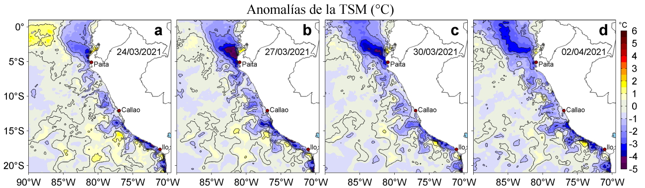
Figura 3. Anomalías de la temperatura superficial del mar (TSM, °C) para los días: a) 24, b) 27 y c) 30 de marzo y d) 02 de abril de 2021. Las anomalías se calcularon respecto de la climatología para el periodo 2007-2016. Datos: OSTIA-UKMO-L4-GLOB-v2.0 (UK Met Office, 2012; Donlon et al, 2012).
