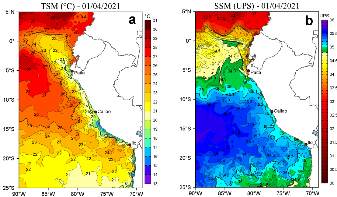
Figura 2. a) Temperatura superficial del mar (TSM, °C) y b) Salinidad superficial del mar (SSM) para el 01 de abril de 2021. Datos: OSTIA-UKMO-L4-GLOB-v2.0 (UK Met Office, 2012; Donlon et al, 2012) disponible en https://podaac.jpl.nasa.gov/dataset/OSTIA-UKMO-L4-GLOB-v2.0 para (a) y Hybrid Coordinate Ocean Model v. GOF5 3.1 (HYCOM; Halliwell et al., 1998; 2000; Bleck, 2001) para (b).
