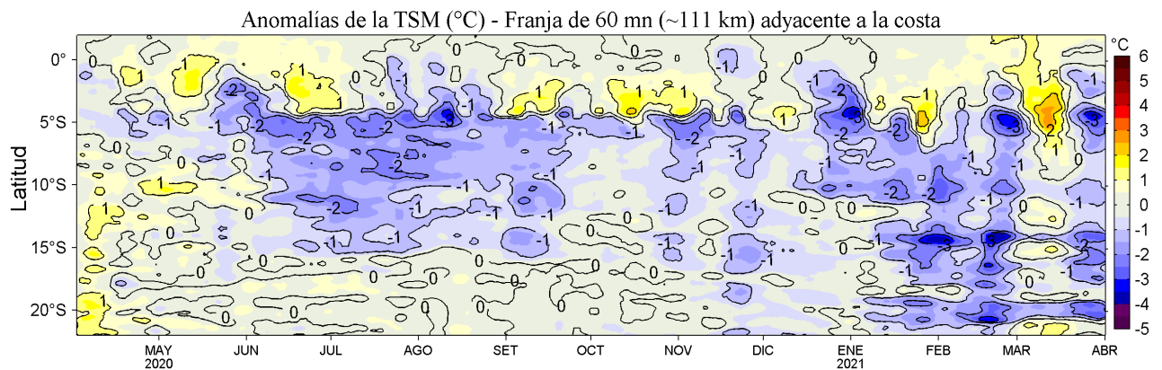
Figura 4. Variación promedio de las anomalías de la temperatura superficial del mar (TSM, °C) para una franja de 60 mn (~111 km) adyacente al litoral peruano para los últimos doce meses al 01 de abril de 2021. Datos: OSTIA-UKMO-L4-GLOB-v2.0 (UK Met. Office, 2012; Donlon et al, 2012) disponible en https://podaac.jpl.nasa.gov/dataset/OSTIA-UKMO-L4-GLOB-v2.0 . Las anomalías se calcularon con respecto al periodo 2007-2016.
