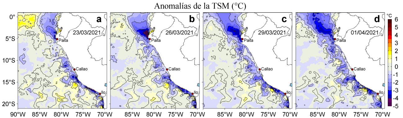
Figura 3. Anomalías de la temperatura superficial del mar (TSM, °C) para los días: a) 23, b) 26 y c) 29 de marzo y d) 01 de abril de 2021. Las anomalías se calcularon respecto de la climatología para el periodo 2007-2016. Datos: OSTIA-UKMO-L4-GLOB-v2.0 (UK Met Office, 2012; Donlon et al, 2012).
