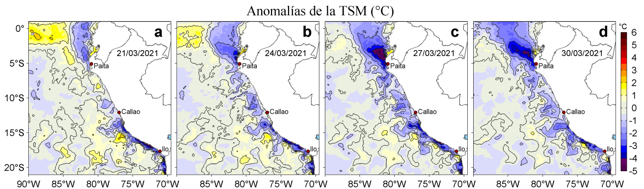
Figura 3. Anomalías de la temperatura superficial del mar (TSM, °C) para los días: a) 21, b) 24, c) 27 y d) 30 de marzo de 2021. Las anomalías se calcularon respecto de la climatología para el periodo 2007-2016. Datos: OSTIA-UKMO-L4-GLOB-v2.0 (UK Met Office, 2012; Donlon et al, 2012).
