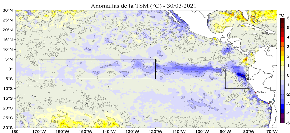
Figura 1. Anomalías de la temperatura superficial del mar (TSM, °C) en el océano Pacífico tropical. Las regiones Niño 3.4 (5°N - 5°S, 170°W - 120°W) y Niño 1+2 (0 - 10°S, 90°W - 80°W) en los sectores central y oriental del océano, respectivamente, están delimitadas con una línea de color negro. Las anomalías se estimaron de acuerdo a la climatología para el periodo 2007-2016. Los datos provienen de OSTIA-UKMO-L4-GLOB-v2.0 (UK Met Office, 2012; Donlon et al, 2012) y están disponibles en https://podaac.jpl.nasa.gov/dataset/OSTIA-UKMO-L4-GLOB-v2.0 .
