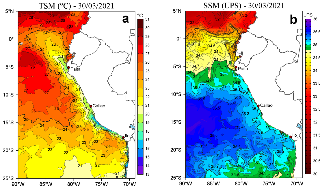
Figura 2. a) Temperatura superficial del mar (TSM, °C) y b) Salinidad superficial del mar (SSM) para el 30 de marzo de 2021. Datos: OSTIA-UKMO-L4-GLOB-v2.0 (UK Met Office, 2012; Donlon et al, 2012) disponible en https://podaac.jpl.nasa.gov/dataset/OSTIA-UKMO-L4-GLOB-v2.0 para (a) y Hybrid Coordinate Ocean Model v. GOF5 3.1 (HYCOM; Halliwell et al., 1998; 2000; Bleck, 2001) para (b).
