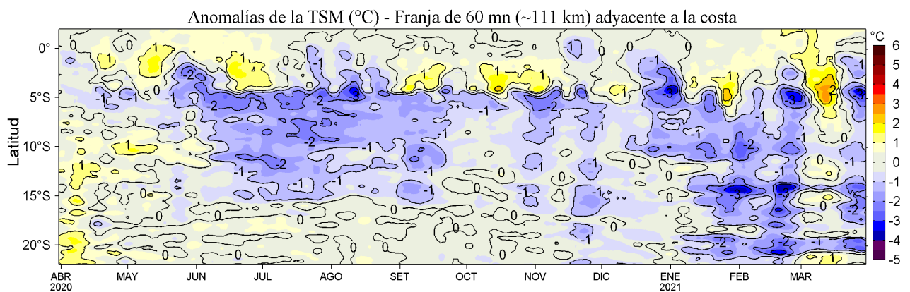
Figura 4. Variación promedio de las anomalías de la temperatura superficial del mar (TSM, °C) para una franja de 60 mn (~111 km) adyacente al litoral peruano para los últimos doce meses al 30 de marzo de 2021. Datos: OSTIA-UKMO-L4-GLOB-v2.0 (UK Met. Office, 2012; Donlon et al, 2012) disponible en https://podaac.jpl.nasa.gov/dataset/OSTIA-UKMO-L4-GLOB-v2.0 . Las anomalías se calcularon con respecto al periodo 2007-2016.
