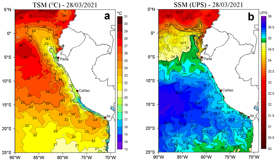
Figura 2. a) Temperatura superficial del mar (TSM, °C) y b) Salinidad superficial del mar (SSM) para el 28 de marzo de 2021. Datos: OSTIA-UKMO-L4-GLOB-v2.0 (UK Met Office, 2012; Donlon et al, 2012) disponible en https://podaac.jpl.nasa.gov/dataset/OSTIA-UKMO-L4-GLOB-v2.0 para (a) y Hybrid Coordinate Ocean Model v. GOF5 3.1 (HYCOM; Halliwell et al., 1998; 2000; Bleck, 2001) para (b).
