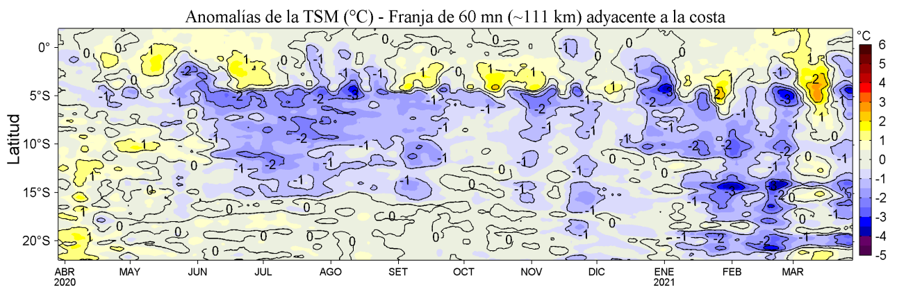
Figura 4. Variación promedio de las anomalías de la temperatura superficial del mar (TSM, °C) para una franja de 60 mn (~111 km) adyacente al litoral peruano para los últimos doce meses al 28 de marzo de 2021. Datos: OSTIA-UKMO-L4-GLOB-v2.0 (UK Met. Office, 2012; Donlon et al, 2012) disponible en https://podaac.jpl.nasa.gov/dataset/OSTIA-UKMO-L4-GLOB-v2.0 . Las anomalías se calcularon con respecto al periodo 2007-2016.
