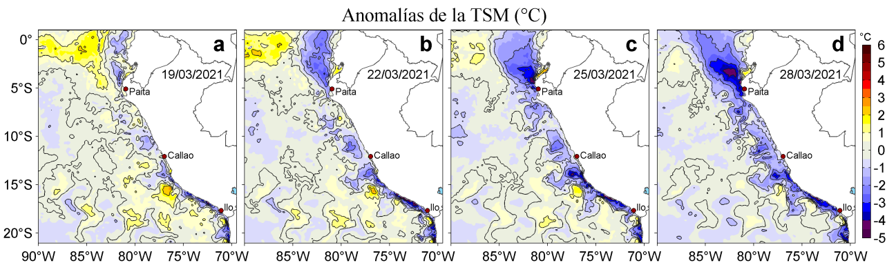
Figura 3. Anomalías de la temperatura superficial del mar (TSM, °C) para los días: a) 19, b) 22, c) 25 y d) 28 de marzo de 2021. Las anomalías se calcularon respecto de la climatología para el periodo 2007-2016. Datos: OSTIA-UKMO-L4-GLOB-v2.0 (UK Met Office, 2012; Donlon et al, 2012).
