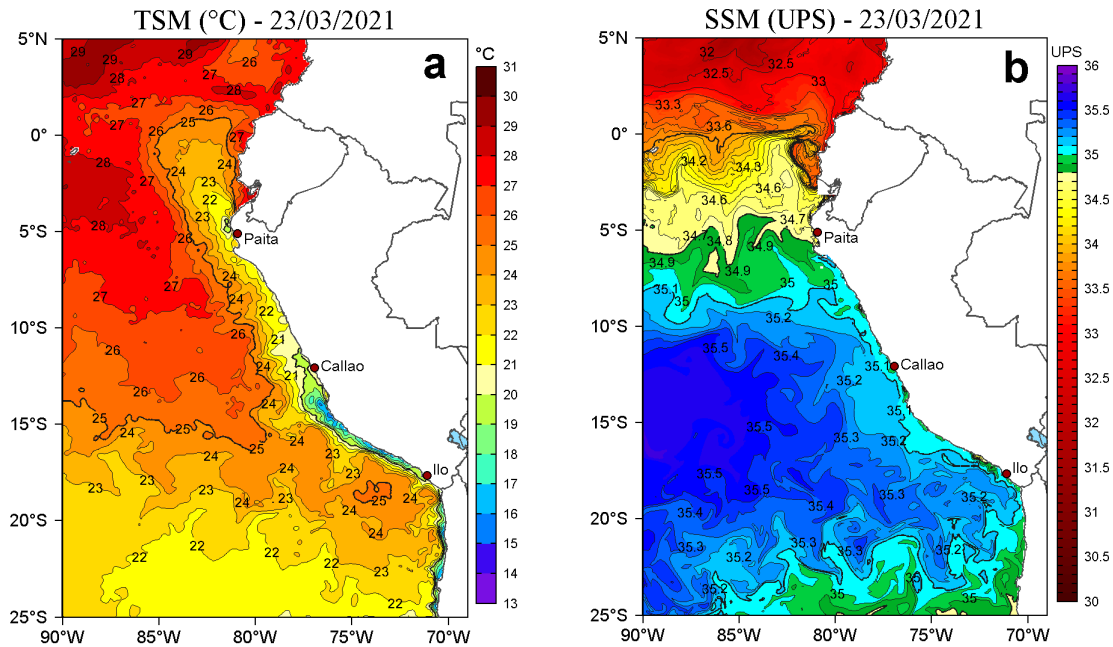
Figura 2. a) Temperatura superficial del mar (TSM, °C) y b) Salinidad superficial del mar (SSM) para el 23 de marzo de 2021. Datos: OSTIA-UKMO-L4-GLOB-v2.0 (UK Met Office, 2012; Donlon et al, 2012) disponible en https://podaac.jpl.nasa.gov/dataset/OSTIA-UKMO-L4-GLOB-v2.0 para (a) y Hybrid Coordinate Ocean Model v. GOF5 3.1 (HYCOM; Halliwell et al., 1998; 2000; Bleck, 2001) para (b).
