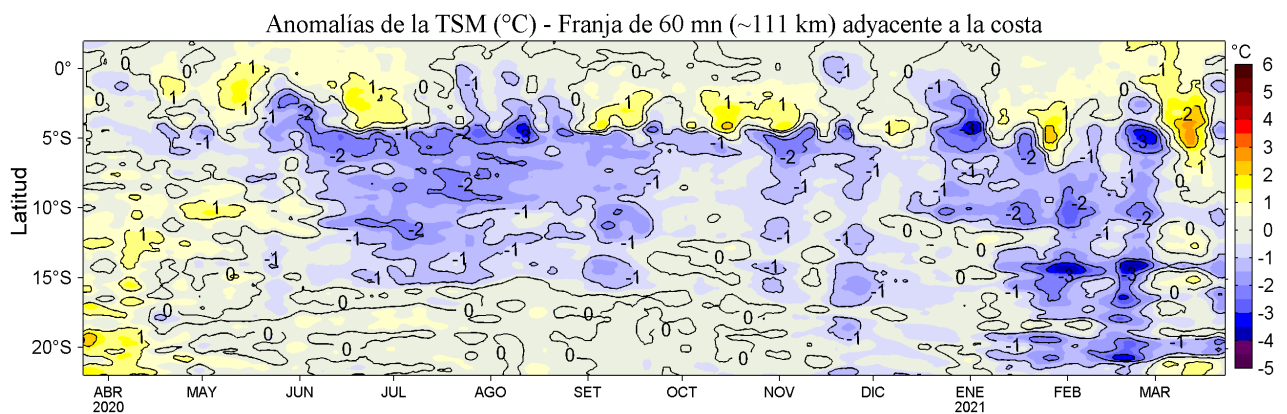
Figura 4. Variación promedio de las anomalías de la temperatura superficial del mar (TSM, °C) para una franja de 60 mn (~111 km) adyacente al litoral peruano para los últimos doce meses al 23 de marzo de 2021. Datos: OSTIA-UKMO-L4-GLOB-v2.0 (UK Met. Office, 2012; Donlon et al, 2012) disponible en https://podaac.jpl.nasa.gov/dataset/OSTIA-UKMO-L4-GLOB-v2.0 . Las anomalías se calcularon con respecto al periodo 2007-2016.
