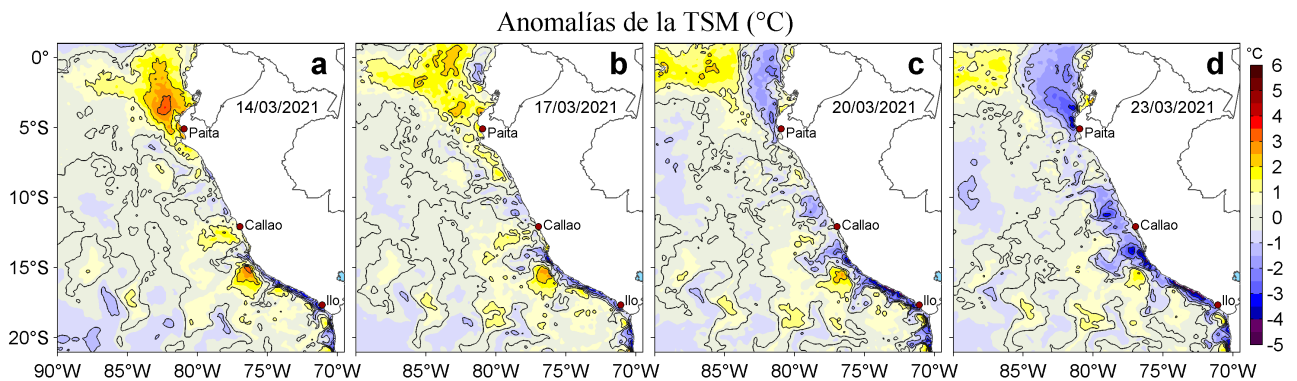
Figura 3. Anomalías de la temperatura superficial del mar (TSM, °C) para los días: a) 14, b) 17, c) 20 y d) 23 de marzo de 2021. Las anomalías se calcularon respecto de la climatología para el periodo 2007-2016. Datos: OSTIA-UKMO-L4-GLOB-v2.0 (UK Met Office, 2012; Donlon et al, 2012).
