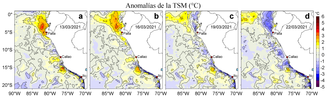
Figura 3. Anomalías de la temperatura superficial del mar (TSM, °C) para los días: a) 13, b) 16, c) 19 y d) 22 de marzo de 2021. Las anomalías se calcularon respecto de la climatología para el periodo 2007-2016. Datos: OSTIA-UKMO-L4-GLOB-v2.0 (UK Met Office, 2012; Donlon et al, 2012).
