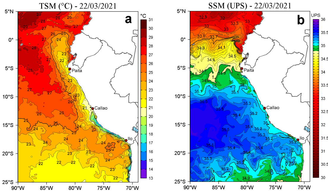
Figura 2. a) Temperatura superficial del mar (TSM, °C) y b) Salinidad superficial del mar (SSM) para el 22 de marzo de 2021. Datos: OSTIA-UKMO-L4-GLOB-v2.0 (UK Met Office, 2012; Donlon et al, 2012) disponible en https://podaac.jpl.nasa.gov/dataset/OSTIA-UKMO-L4-GLOB-v2.0 para (a) y Hybrid Coordinate Ocean Model v. GOFS 3.1 (HYCOM; Halliwell et al., 1998; 2000; Bleck, 2001) para (b).
