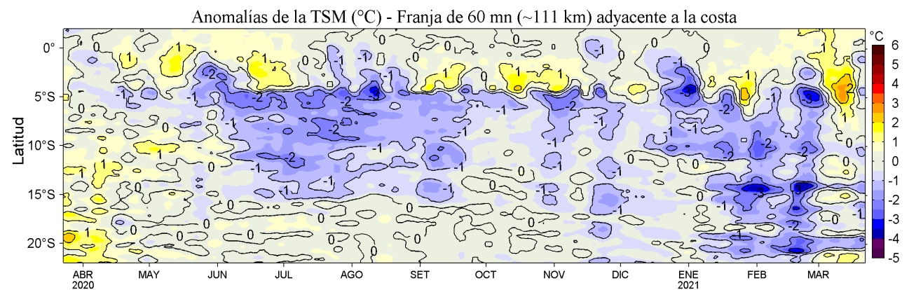
Figura 4. Variación promedio de las anomalías de la temperatura superficial del mar (TSM, °C) para una franja de 60 mn (~111 km) adyacente al litoral peruano para los últimos doce meses al 22 de marzo de 2021. Datos: OSTIA-UKMO-L4-GLOB-v2.0 (UK Met. Office, 2012; Donlon et al, 2012) disponible en https://podaac.jpl.nasa.gov/dataset/OSTIA-UKMO-L4-GLOB-v2.0 . Las anomalías se calcularon con respecto al periodo 2007-2016.
