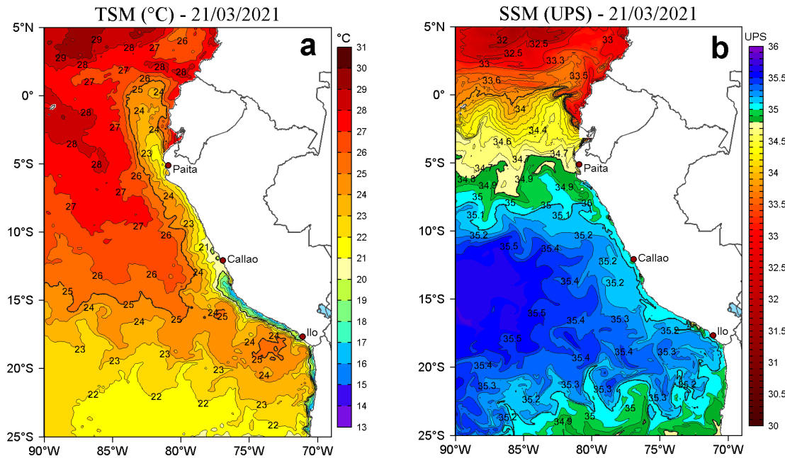
Figura 2. a) Temperatura superficial del mar (TSM, °C) y b) Salinidad superficial del mar (SSM) para el 21 de marzo de 2021. Datos: OSTIA-UKMO-L4-GLOB-v2.0 (UK Met Office, 2012; Donlon et al, 2012) disponible en https://podaac.jpl.nasa.gov/dataset/OSTIA-UKMO-L4-GLOB-v2.0 para (a) y Hybrid Coordinate Ocean Model v. GOFS 3.1 (HYCOM; Halliwell et al., 1998; 2000; Bleck, 2001) para (b).
