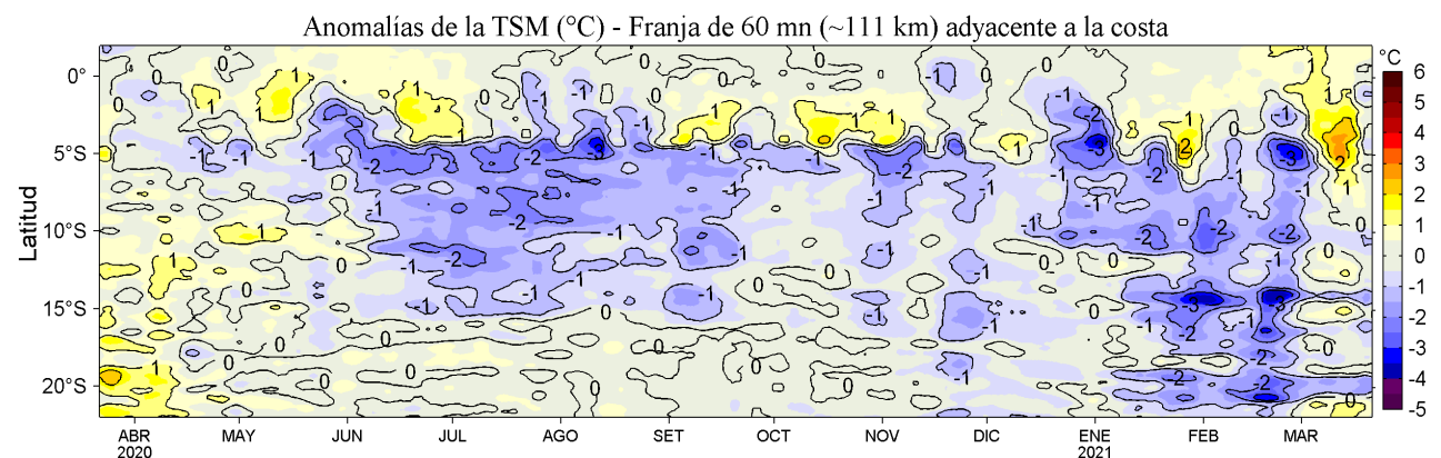
Figura 4. Variación promedio de las anomalías de la temperatura superficial del mar (TSM, °C) para una franja de 60 mn (~111 km) adyacente al litoral peruano para los últimos doce meses al 21 de marzo de 2021. Datos: OSTIA-UKMO-L4-GLOB-v2.0 (UK Met. Office, 2012; Donlon et al, 2012) disponible en https://podaac.jpl.nasa.gov/dataset/OSTIA-UKMO-L4-GLOB-v2.0 . Las anomalías se calcularon con respecto al periodo 2007-2016.
