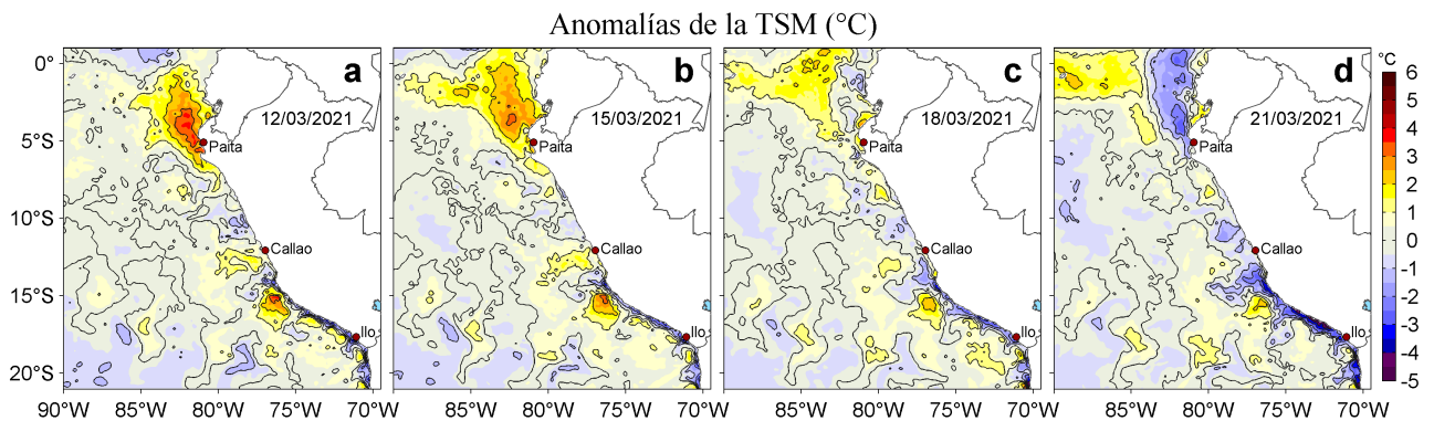
Figura 3. Anomalías de la temperatura superficial del mar (TSM, °C) para los días: a) 12, b) 15, c) 18 y d) 21 de marzo de 2021. Las anomalías se calcularon respecto de la climatología para el periodo 2007-2016. Datos: OSTIA-UKMO-L4-GLOB-v2.0 (UK Met Office, 2012; Donlon et al, 2012).
