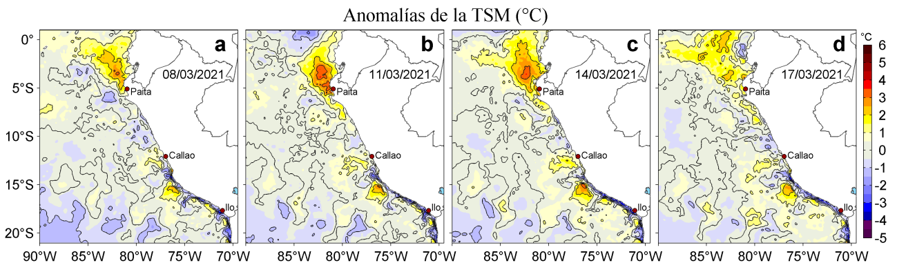
Figura 3. Anomalías de la temperatura superficial del mar (TSM, °C) para los días: a) 08, b) 11, c) 14 y d) 17 de marzo de 2021. Las anomalías se calcularon respecto de la climatología para el periodo 2007-2016. Datos: OSTIA-UKMO-L4-GLOB-v2.0 (UK Met Office, 2012; Donlon et al, 2012).
