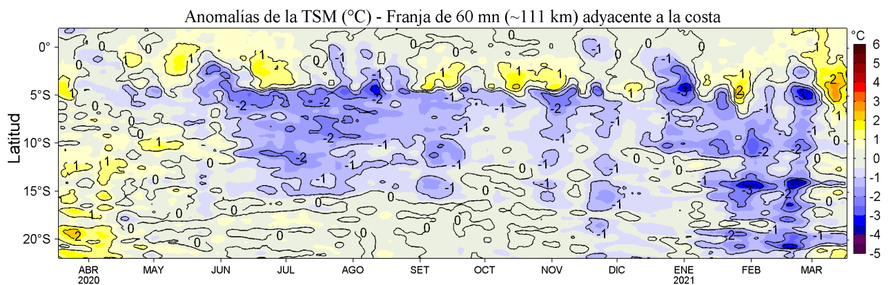
Figura 4. Variación promedio de las anomalías de la temperatura superficial del mar (TSM, °C) para una franja de 60 mn (~111 km) adyacente al litoral peruano para los últimos doce meses al 17 de marzo de 2021. Datos: OSTIA-UKMO-L4-GLOB-v2.0 (UK Met. Office, 2012; Donlon et al, 2012) disponible en https://podaac.jpl.nasa.gov/dataset/OSTIA-UKMO-L4-GLOB-v2.0 . Las anomalías se calcularon con respecto al periodo 2007-2016.
