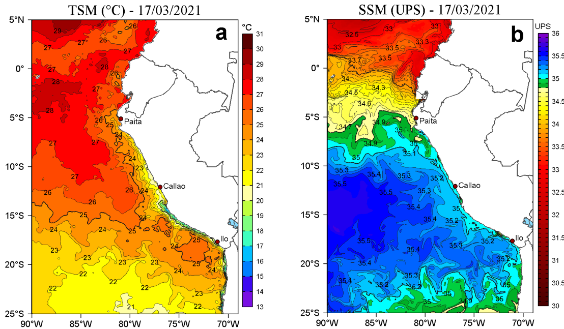
Figura 2. a) Temperatura superficial del mar (TSM, °C) y b) Salinidad superficial del mar (SSM) para el 17 de marzo de 2021. Datos: OSTIA-UKMO-L4-GLOB-v2.0 (UK Met Office, 2012; Donlon et al, 2012) disponible en https://podaac.jpl.nasa.gov/dataset/OSTIA-UKMO-L4-GLOB-v2.0 para (a) y Hybrid Coordinate Ocean Model v. GOFS 3.1 (HYCOM; Halliwell et al., 1998; 2000; Bleck, 2001) para (b).
