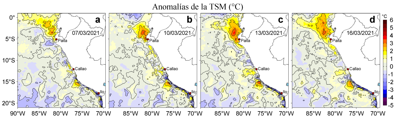
Figura 3. Anomalías de la temperatura superficial del mar (TSM, °C) para los días: a) 07, b) 10, c) 13 y d) 16 de marzo de 2021. Las anomalías se calcularon respecto de la climatología para el periodo 2007-2016. Datos: OSTIA-UKMO-L4-GLOB-v2.0 (UK Met Office, 2012; Donlon et al, 2012).
