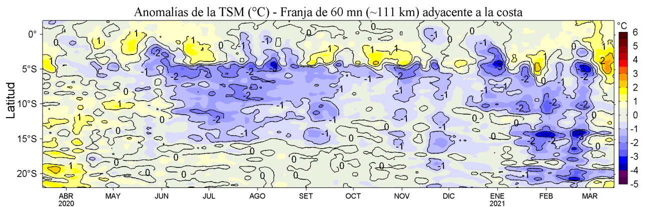
Figura 4. Variación promedio de las anomalías de la temperatura superficial del mar (TSM, °C) para una franja de 60 mn (~111 km) adyacente al litoral peruano para los últimos doce meses al 16 de marzo de 2021. Datos: OSTIA-UKMO-L4-GLOB-v2.0 (UK Met. Office, 2012; Donlon et al, 2012) disponible en https://podaac.jpl.nasa.gov/dataset/OSTIA-UKMO-L4-GLOB-v2.0 . Las anomalías se calcularon con respecto al periodo 2007-2016.
