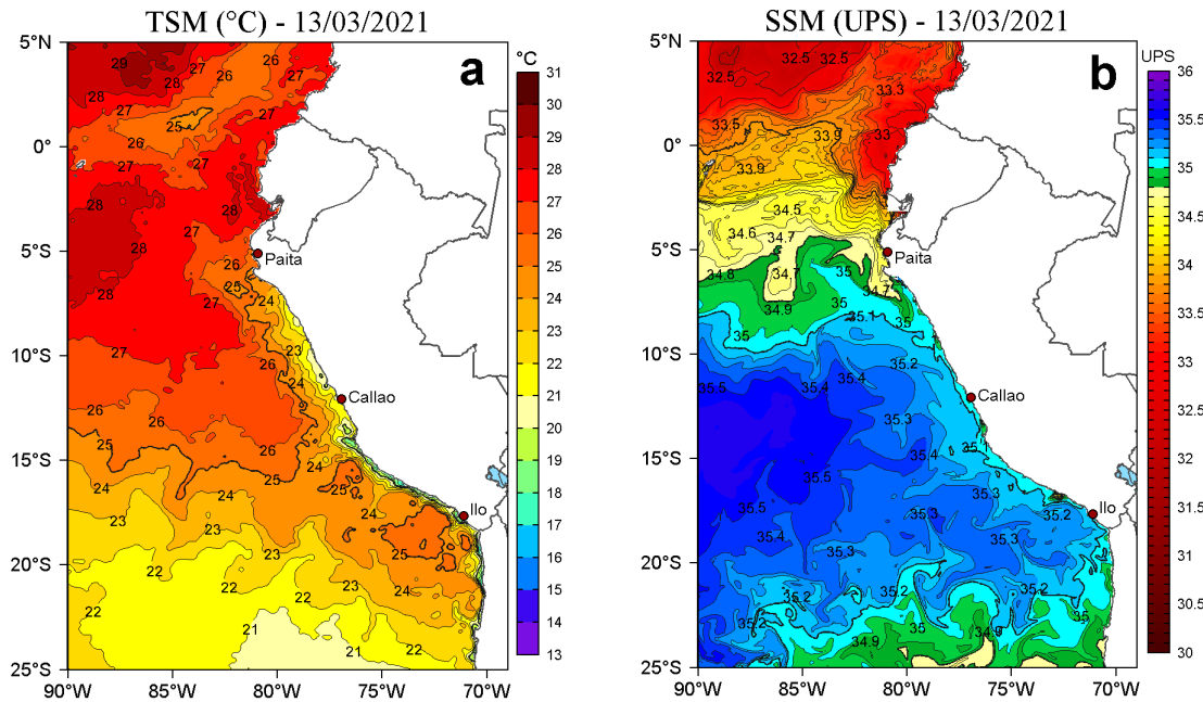
Figura 2. a) Temperatura superficial del mar (TSM, °C) y b) Salinidad superficial del mar (SSM) para el 13 de marzo de 2021. Datos: OSTIA-UKMO-L4-GLOB-v2.0 (UK Met Office, 2012; Donlon et al, 2012) disponible en https://podaac.jpl.nasa.gov/dataset/OSTIA-UKMO-L4-GLOB-v2.0 para (a) y Hybrid Coordinate Ocean Model v. GOFS 3.1 (HYCOM; Halliwell et al., 1998; 2000; Bleck, 2001) para (b).
