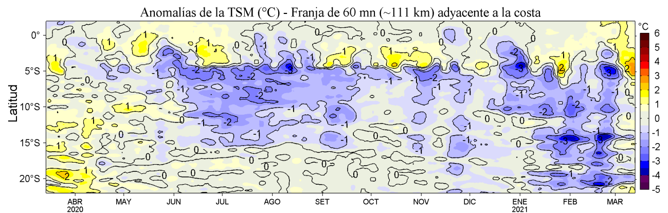
Figura 4. Variación promedio de las anomalías de la temperatura superficial del mar (TSM, °C) para una franja de 60 mn (~111 km) adyacente al litoral peruano para los últimos doce meses al 13 de marzo de 2021. Datos: OSTIA-UKMO-L4-GLOB-v2.0 (UK Met. Office, 2012; Donlon et al, 2012) disponible en https://podaac.jpl.nasa.gov/dataset/OSTIA-UKMO-L4-GLOB-v2.0 . Las anomalías se calcularon con respecto al periodo 2007-2016.
