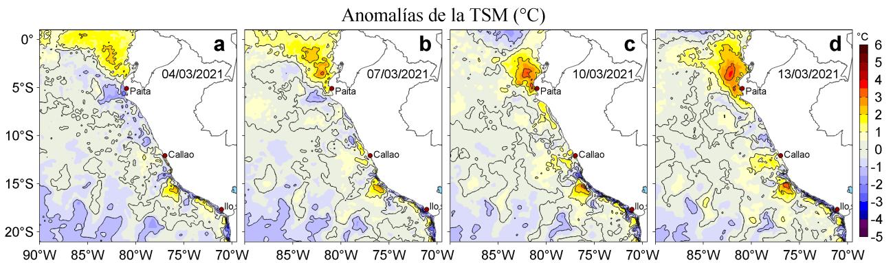
Figura 3. Anomalías de la temperatura superficial del mar (TSM, °C) para los días: a) 04, b) 07, c) 10 y d) 13 de marzo de 2021. Las anomalías se calcularon respecto de la climatología para el periodo 2007-2016. Datos: OSTIA-UKMO-L4-GLOB-v2.0 (UK Met Office, 2012; Donlon et al, 2012).
