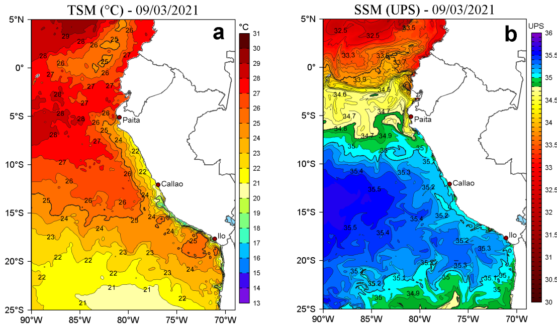
Figura 2. a) Temperatura superficial del mar (TSM, °C) y b) Salinidad superficial del mar (SSM) para el 09 de marzo de 2021. Datos: OSTIA-UKMO-L4-GLOB-v2.0 (UK Met Office, 2012; Donlon et al, 2012) disponible en https://podaac.jpl.nasa.gov/dataset/OSTIA-UKMO-L4-GLOB-v2.0 para (a) y Hybrid Coordinate Ocean Model v. GOFS 3.1 (HYCOM; Halliwell et al., 1998; 2000; Bleck, 2001) para (b).
