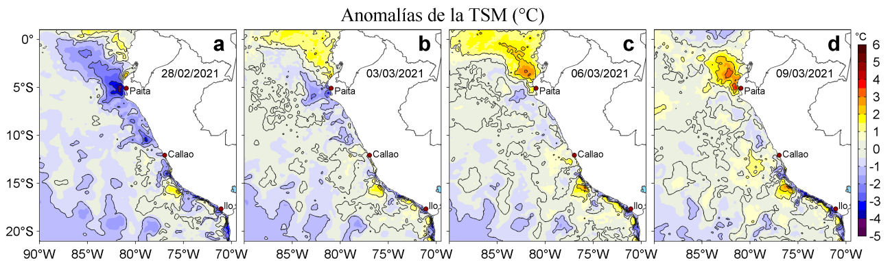
Figura 3. Anomalías de la temperatura superficial del mar (TSM, °C) para los días: a) 28 de febrero, b) 03, c) 06 y d) 09 de marzo de 2021. Las anomalías se calcularon respecto de la climatología para el periodo 2007-2016. Datos: OSTIA-UKMO-L4-GLOB-v2.0 (UK Met Office, 2012; Donlon et al, 2012).
