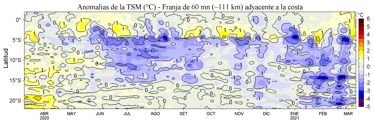
Figura 4. Variación promedio de las anomalías de la temperatura superficial del mar (TSM, °C) para una franja de 60 mn (~111 km) adyacente al litoral peruano para los últimos doce meses al 09 de marzo de 2021. Datos: OSTIA-UKMO-L4-GLOB-v2.0 (UK Met. Office, 2012; Donlon et al, 2012) disponible en https://podaac.jpl.nasa.gov/dataset/OSTIA-UKMO-L4-GLOB-v2.0 . Las anomalías se calcularon con respecto al periodo 2007-2016.
