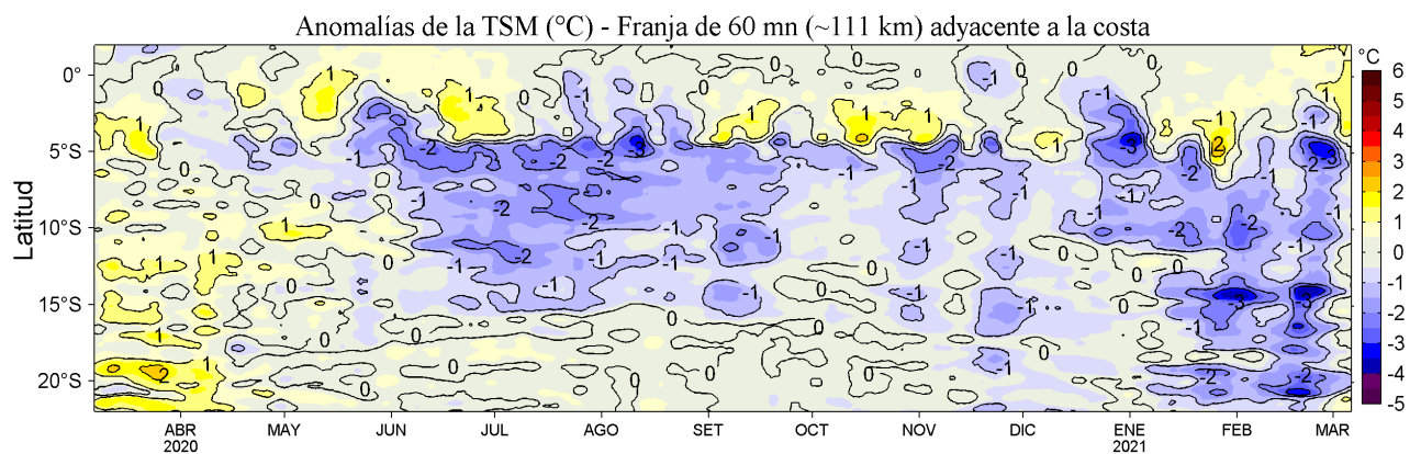
Figura 4. Variación promedio de las anomalías de la temperatura superficial del mar (TSM, °C) para una franja de 60 mn (~111 km) adyacente al litoral peruano para los últimos doce meses al 06 de marzo de 2021. Datos: OSTIA-UKMO-L4-GLOB-v2.0 (UK Met. Office, 2012; Donlon et al, 2012) disponible en https://podaac.jpl.nasa.gov/dataset/OSTIA-UKMO-L4-GLOB-v2.0 . Las anomalías se calcularon con respecto al periodo 2007-2016.
