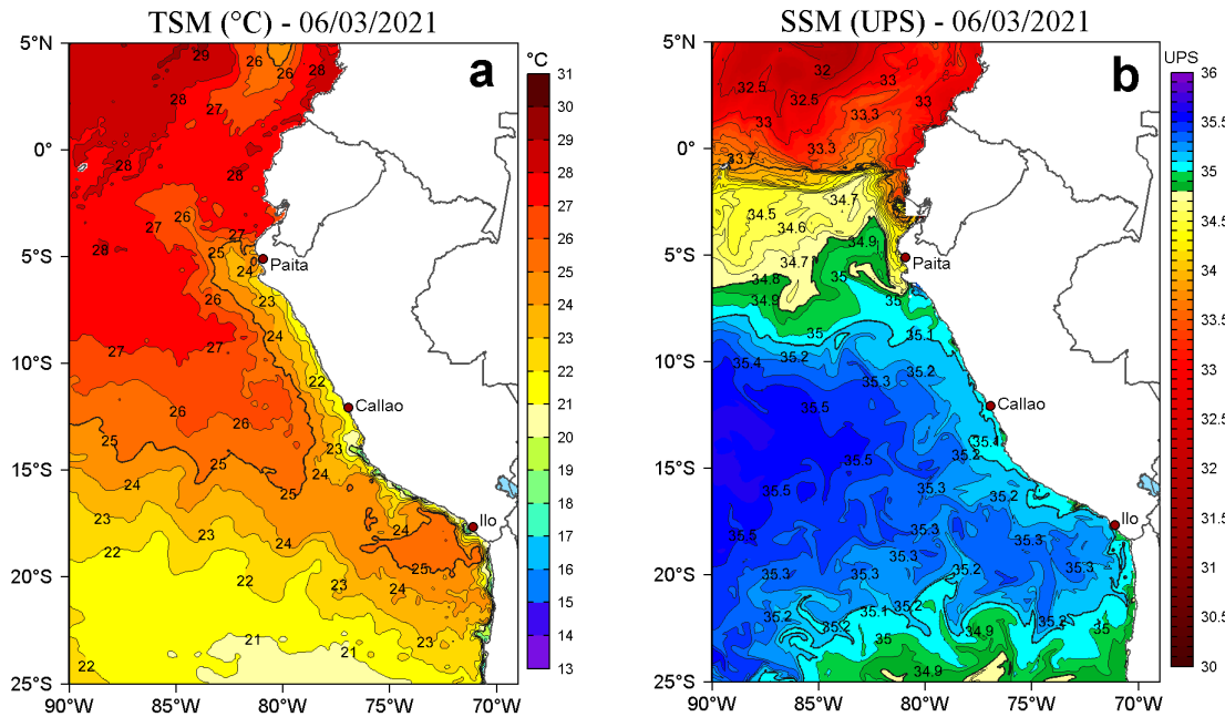
Figura 2. a) Temperatura superficial del mar (TSM, °C) y b) Salinidad superficial del mar (SSM) para el 06 de marzo de 2021. Datos: OSTIA-UKMO-L4-GLOB-v2.0 (UK Met Office, 2012; Donlon et al, 2012) disponible en https://podaac.jpl.nasa.gov/dataset/OSTIA-UKMO-L4-GLOB-v2.0 para (a) y Hybrid Coordinate Ocean Model v. GOF5 3.1 (HYCOM; Halliwell et al., 1998; 2000; Bleck, 2001) para (b).
