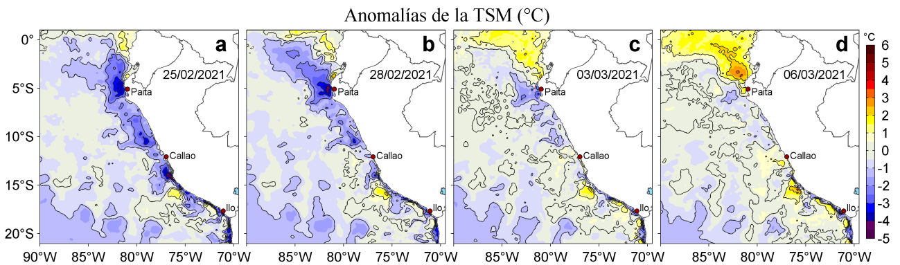
Figura 3. Anomalías de la temperatura superficial del mar (TSM, °C) para los días: a) 25 y b) 28 de febrero, c) 03 y d) 06 de marzo de 2021. Las anomalías se calcularon respecto de la climatología para el periodo 2007-2016. Datos: OSTIA-UKMO-L4-GLOB-v2.0 (UK Met Office, 2012; Donlon et al, 2012).
