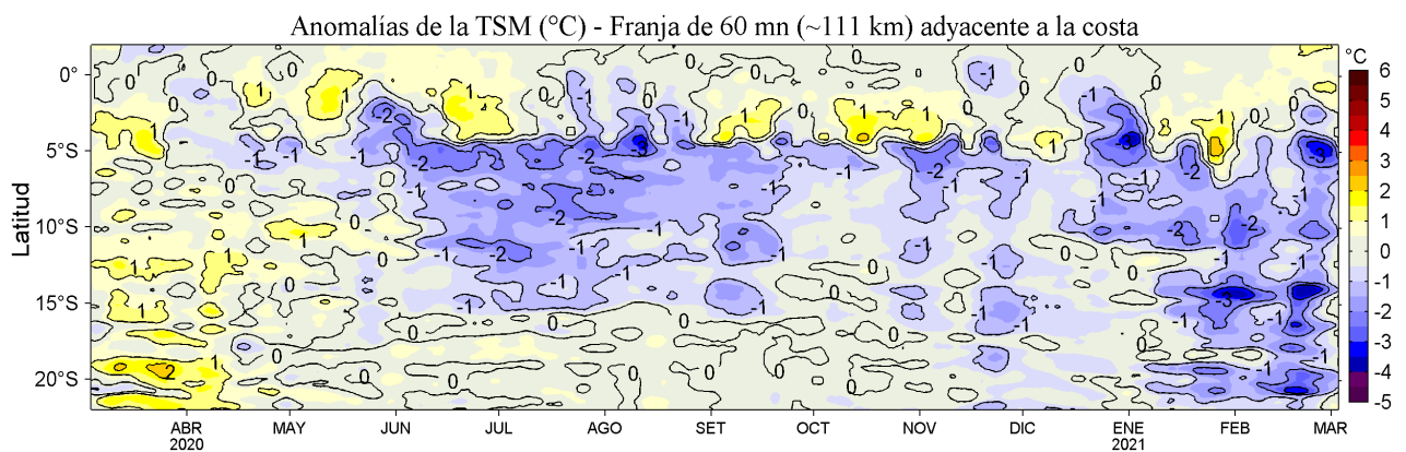
Figura 4. Variación promedio de las anomalías de la temperatura superficial del mar (TSM, °C) para una franja de 60 mn (~111 km) adyacente al litoral peruano para los últimos doce meses al 03 de marzo de 2021. Datos: OSTIA-UKMO-L4-GLOB-v2.0 (UK Met. Office, 2012; Donlon et al, 2012) disponible en https://podaac.jpl.nasa.gov/dataset/OSTIA-UKMO-L4-GLOB-v2.0 . Las anomalías se calcularon con respecto al periodo 2007-2016.
