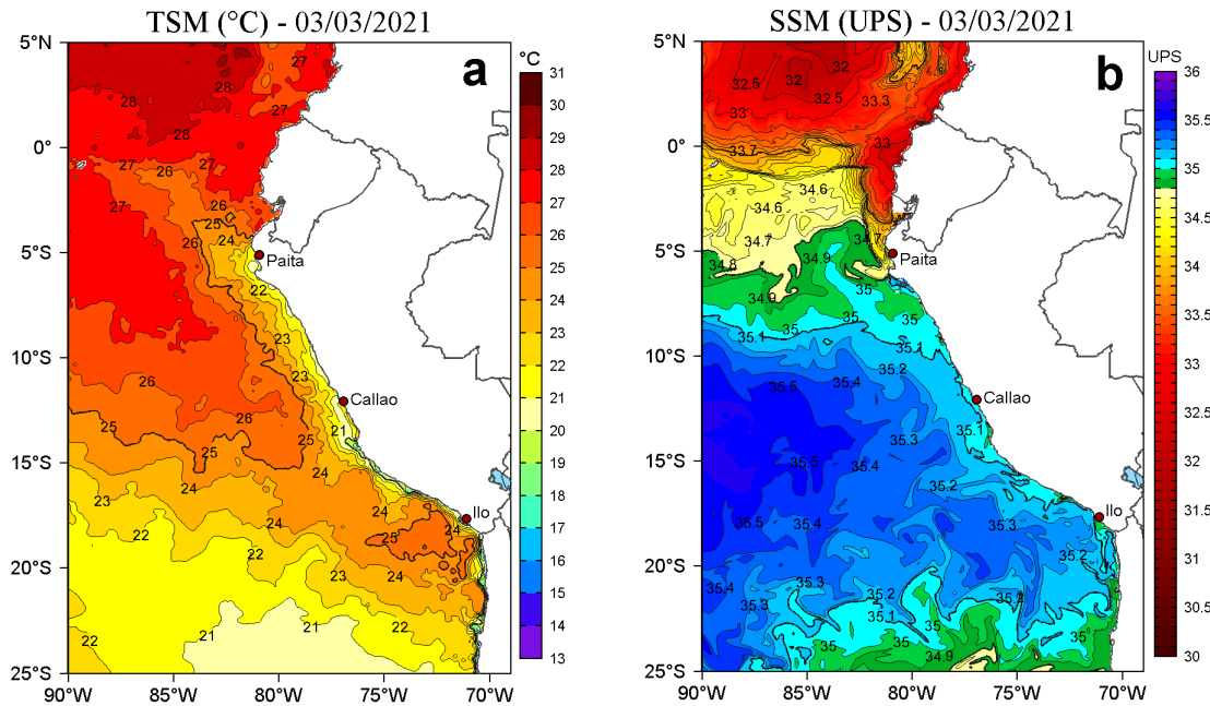
Figura 2. a) Temperatura superficial del mar (TSM, °C) y b) Salinidad superficial del mar (SSM) para el 03 de marzo de 2021. Datos: OSTIA-UKMO-L4-GLOB-v2.0 (UK Met Office, 2012; Donlon et al, 2012) disponible en https://podaac.jpl.nasa.gov/dataset/OSTIA-UKMO-L4-GLOB-v2.0 para (a) y Hybrid Coordinate Ocean Model v. GOFS 3.1 (HYCOM; Halliwell et al., 1998; 2000; Bleck, 2001) para (b).
