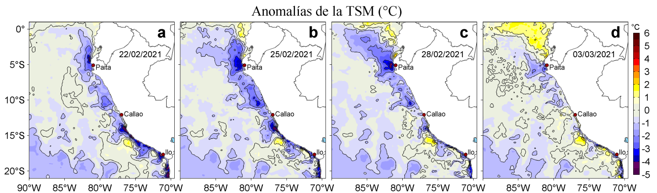
Figura 3. Anomalías de la temperatura superficial del mar (TSM, °C) para los días: a) 22, b) 25 y c) 28 de febrero y d) 03 de marzo de 2021. Las anomalías se calcularon respecto de la climatología para el periodo 2007-2016. Datos: OSTIA-UKMO-L4-GLOB-v2.0 (UK Met Office, 2012; Donlon et al, 2012).
